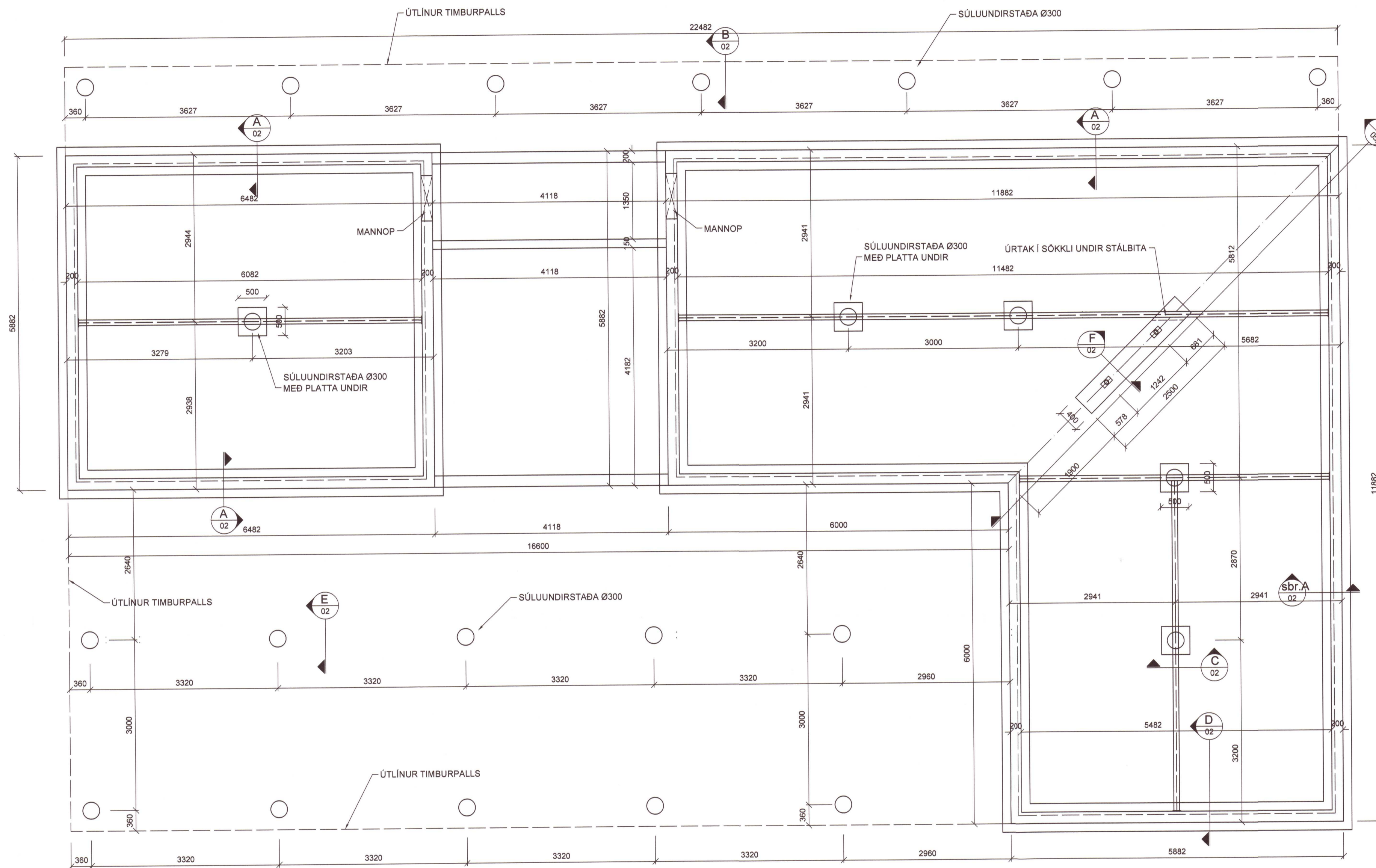
GRUNNMYND SÖKKLA 1:50
