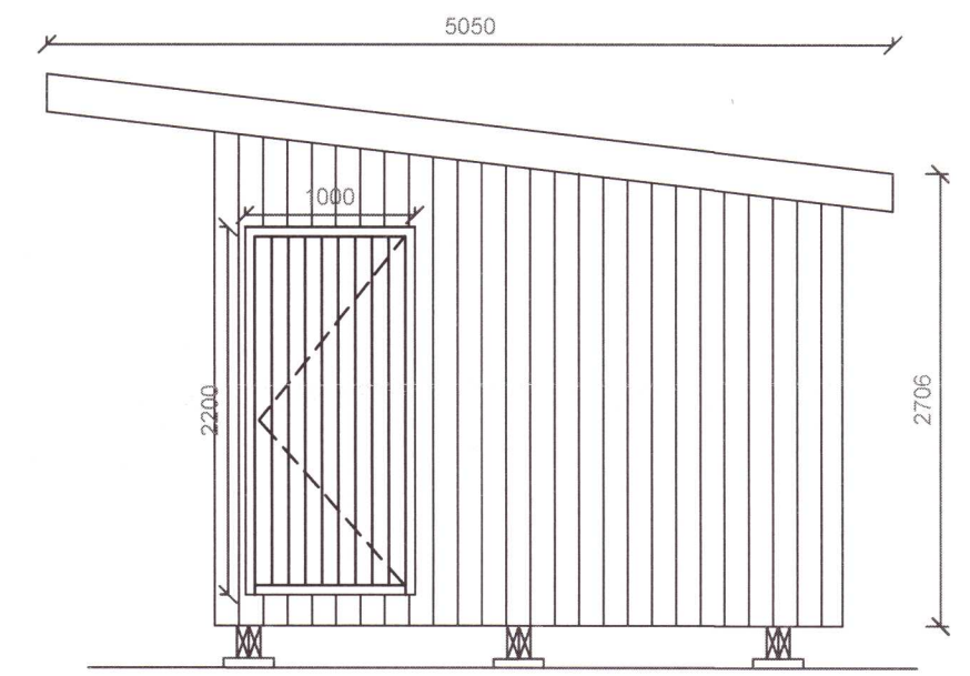
ÚTLIT SUÐAUSTUR 1:50
