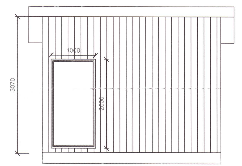
ÚTLIT SUÐVESTUR 1:50
