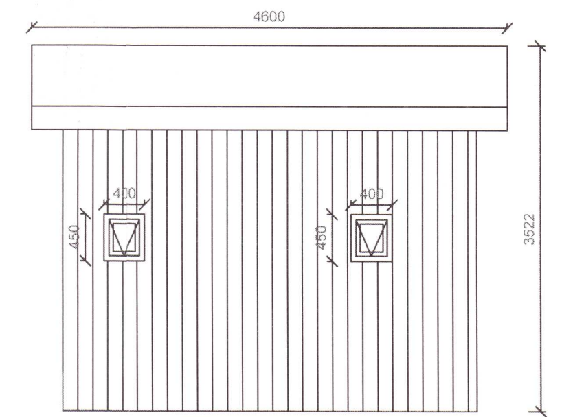
ÚTLIT NORÐAUSTUR 1:50
