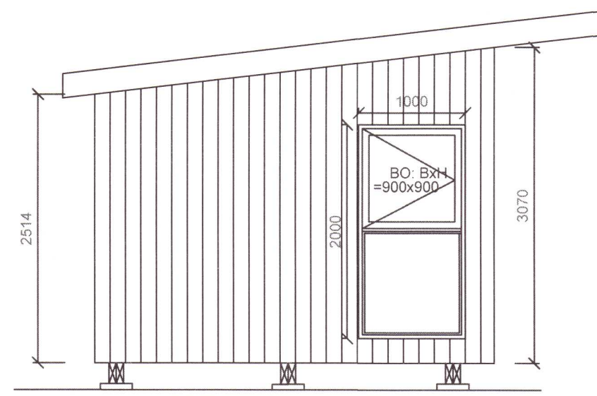
ÚTLIT NORÐVESTUR 1:50
