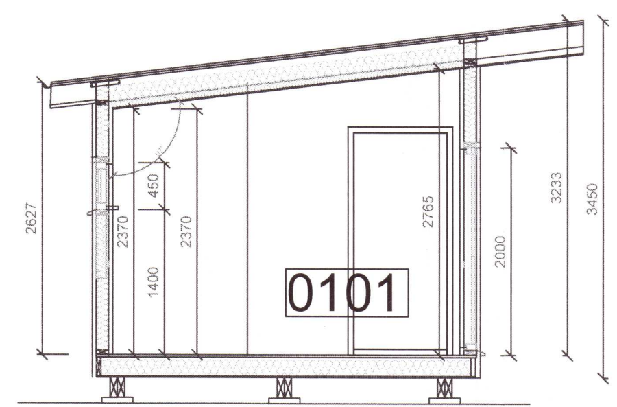
SNÍÐ A-A 1:50
