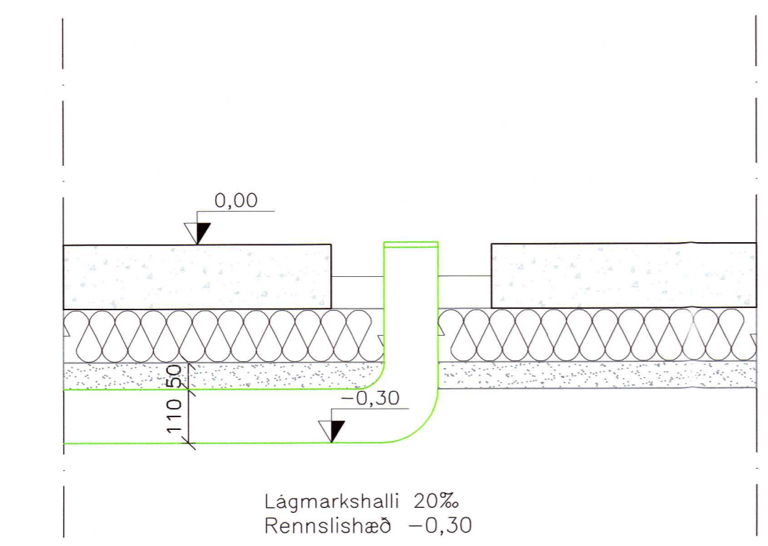
A Snið - Stútar í gólfi, almennt Mkv: 1:10
