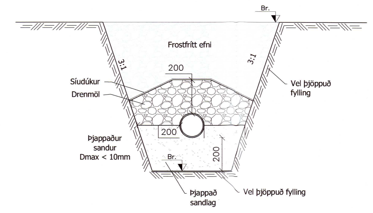
C Snið - Dren- og regnvatnslagnir, almennt skurðsnið Mkv: 1:10
