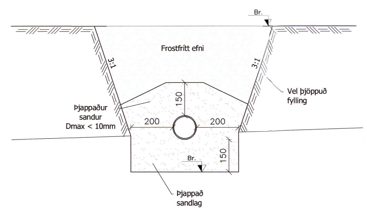
B Snið - Fráveitulagnir, almennt skurðsnið Mkv: 1:10
