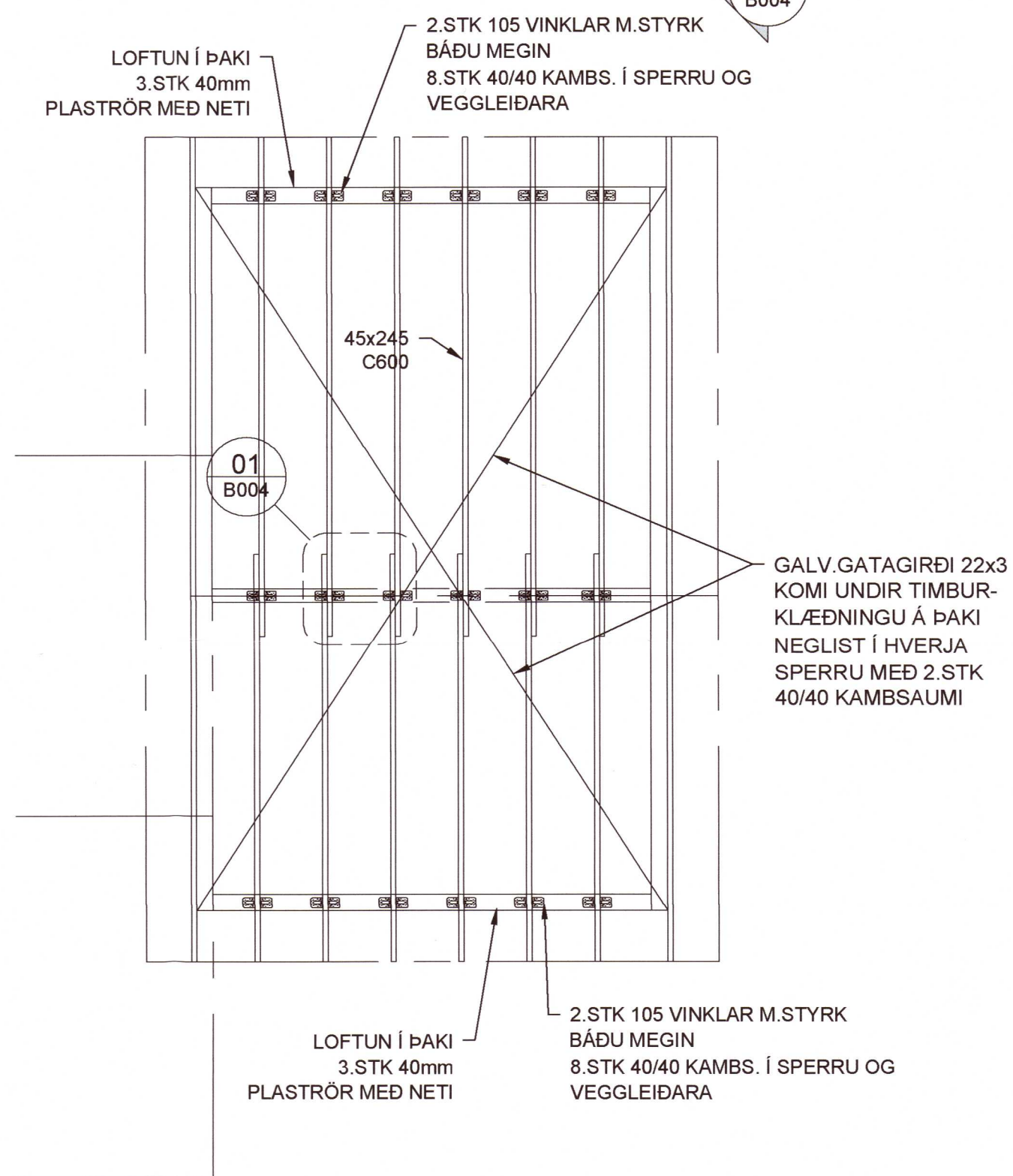
GRUNNMYND - ÞAKVIRKI 1:50 (A1)
