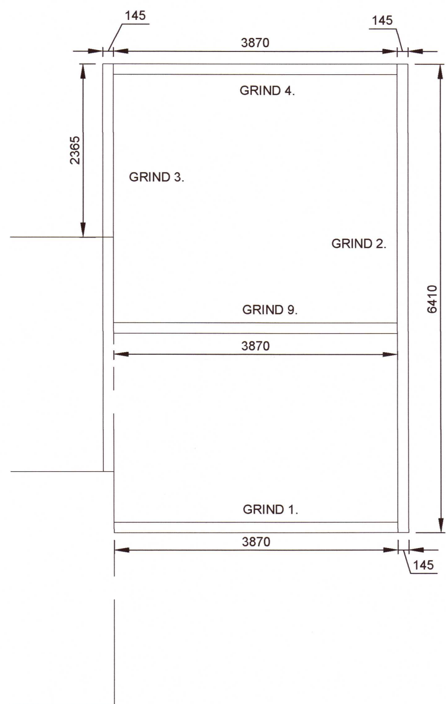
GRUNNMYND - BURÐARVEGGIR 1:50 (A1)
