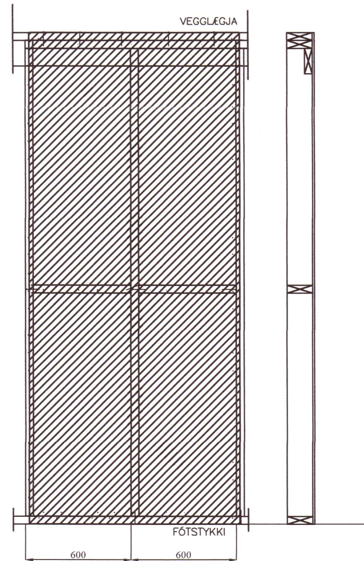
UPPBYGGING ÚTVEGGJA Mkv. 1:20
