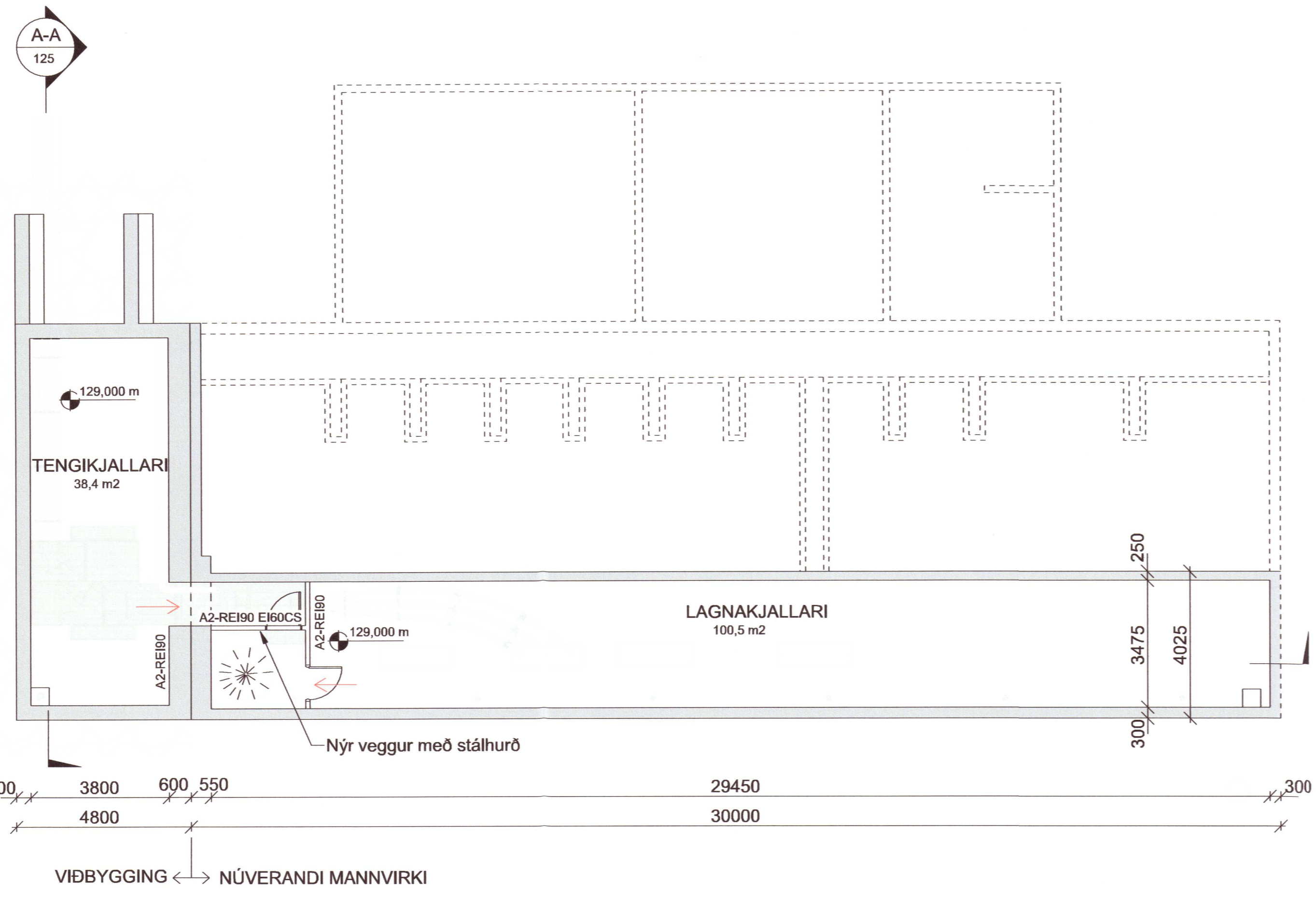
Tengivirki - Kjallari - Grunnmynd gk. 129,00 1 : 100
