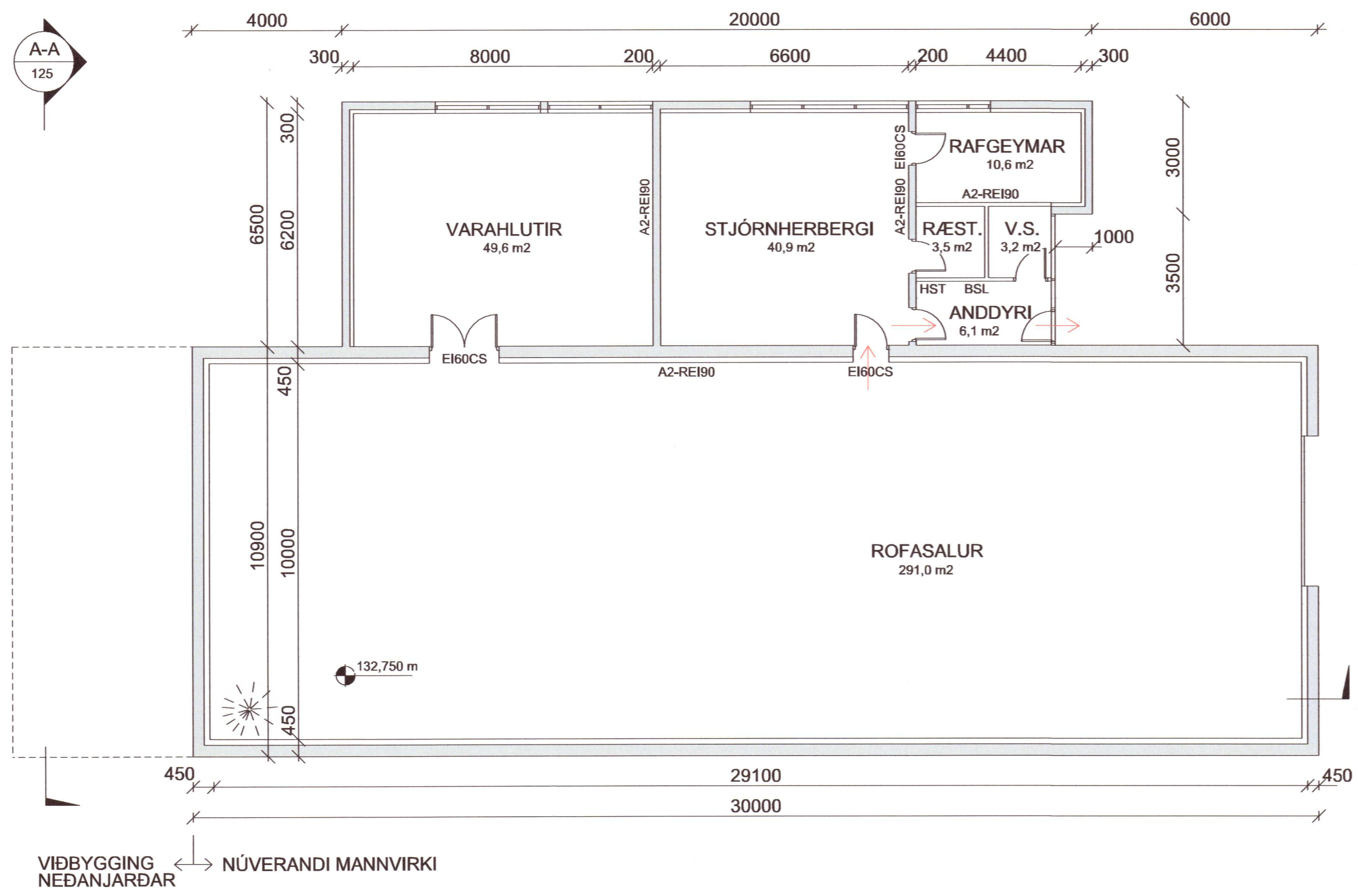
Tengivirki - Grunnmynd gk. 132,75 1 : 100
