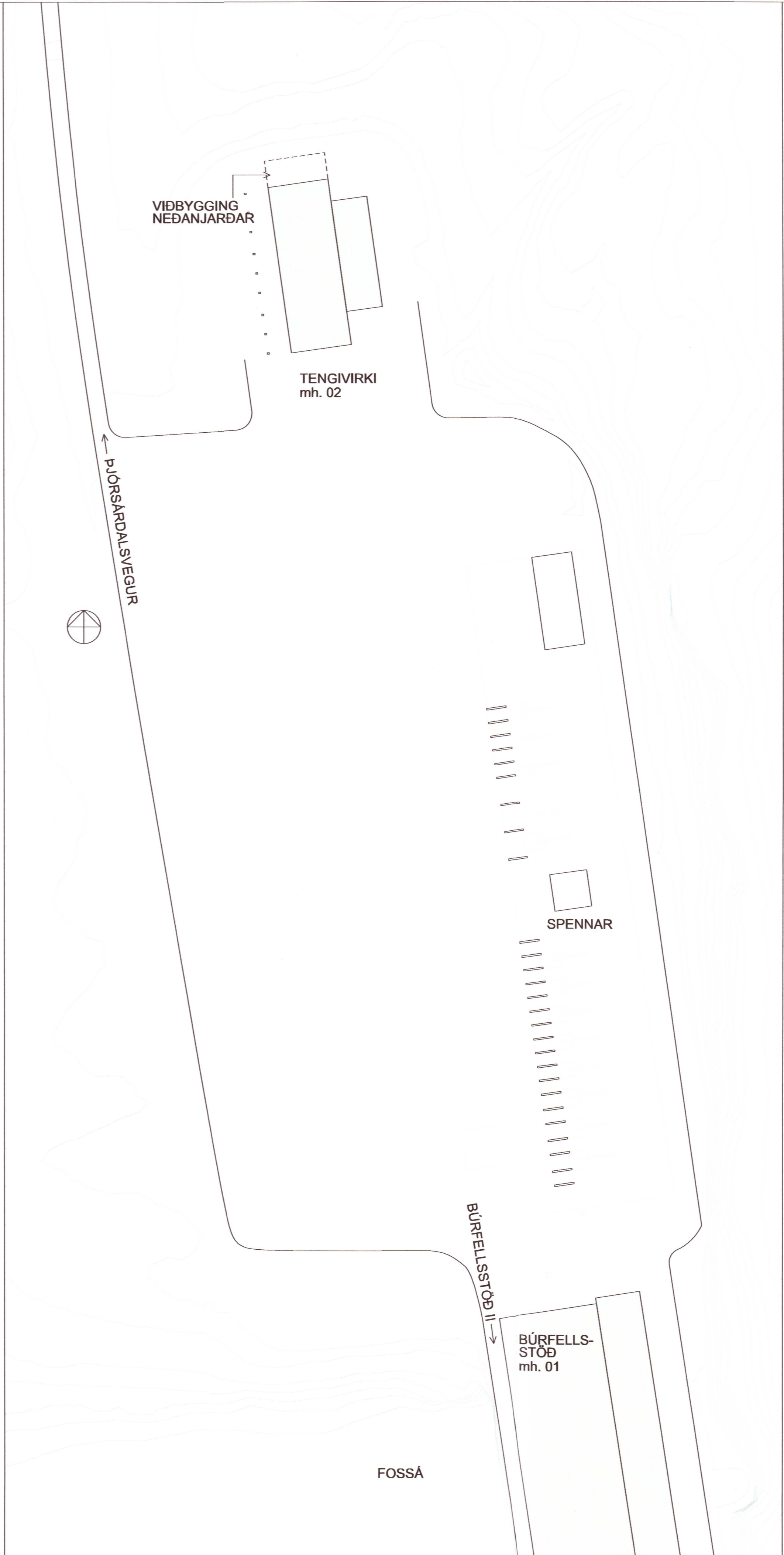
Tengivirki - Afstöðumynd 1 : 500
