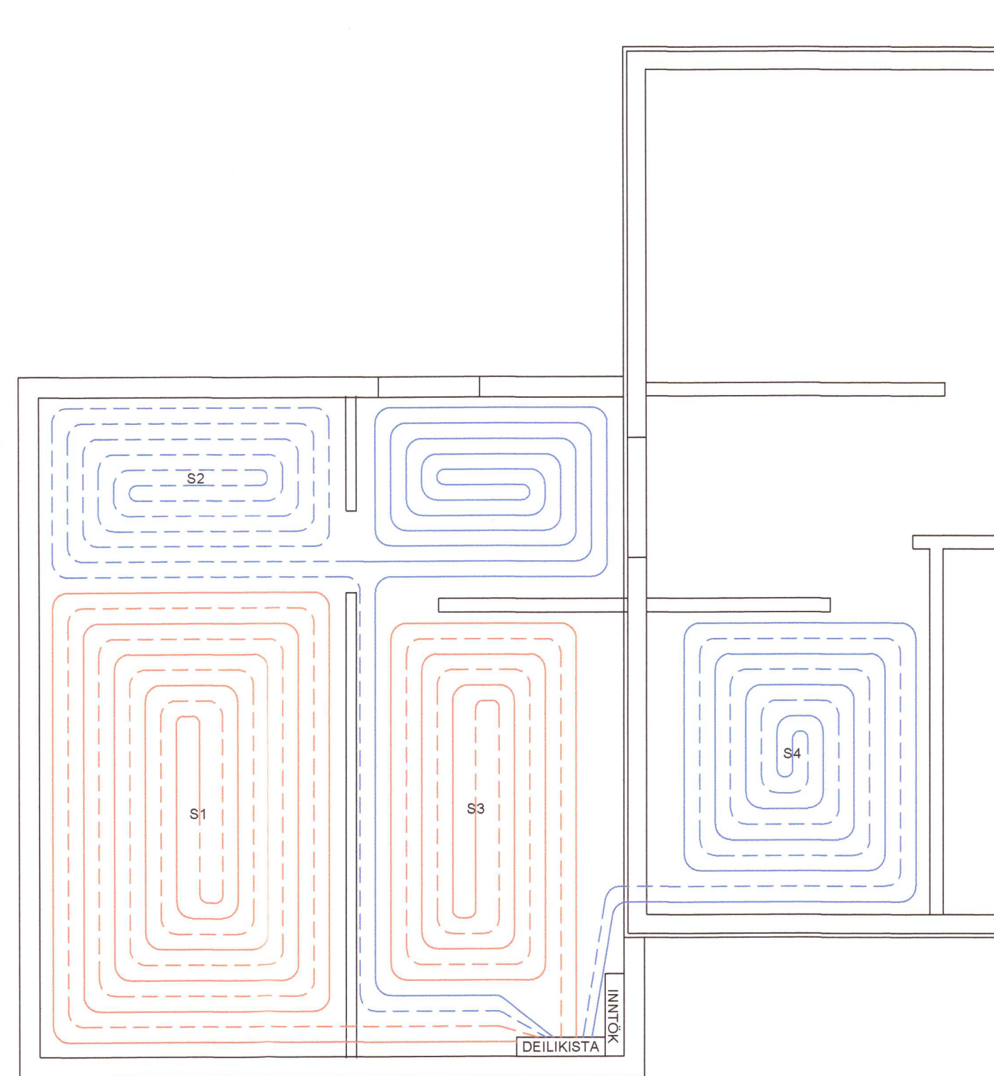
GRUNNMYND Mkv. 1:50
