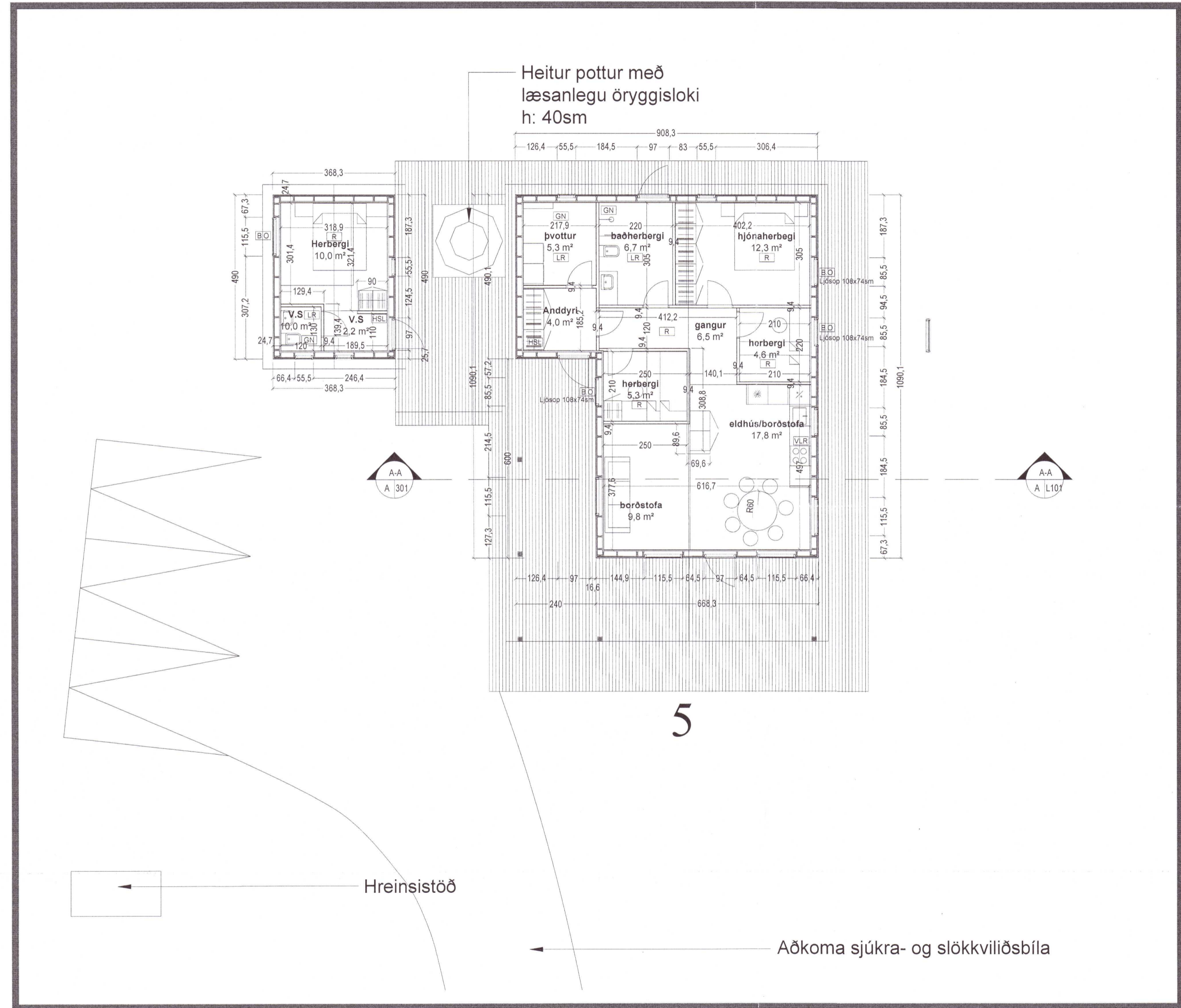
Grunnmynd Mkv. 1:100
