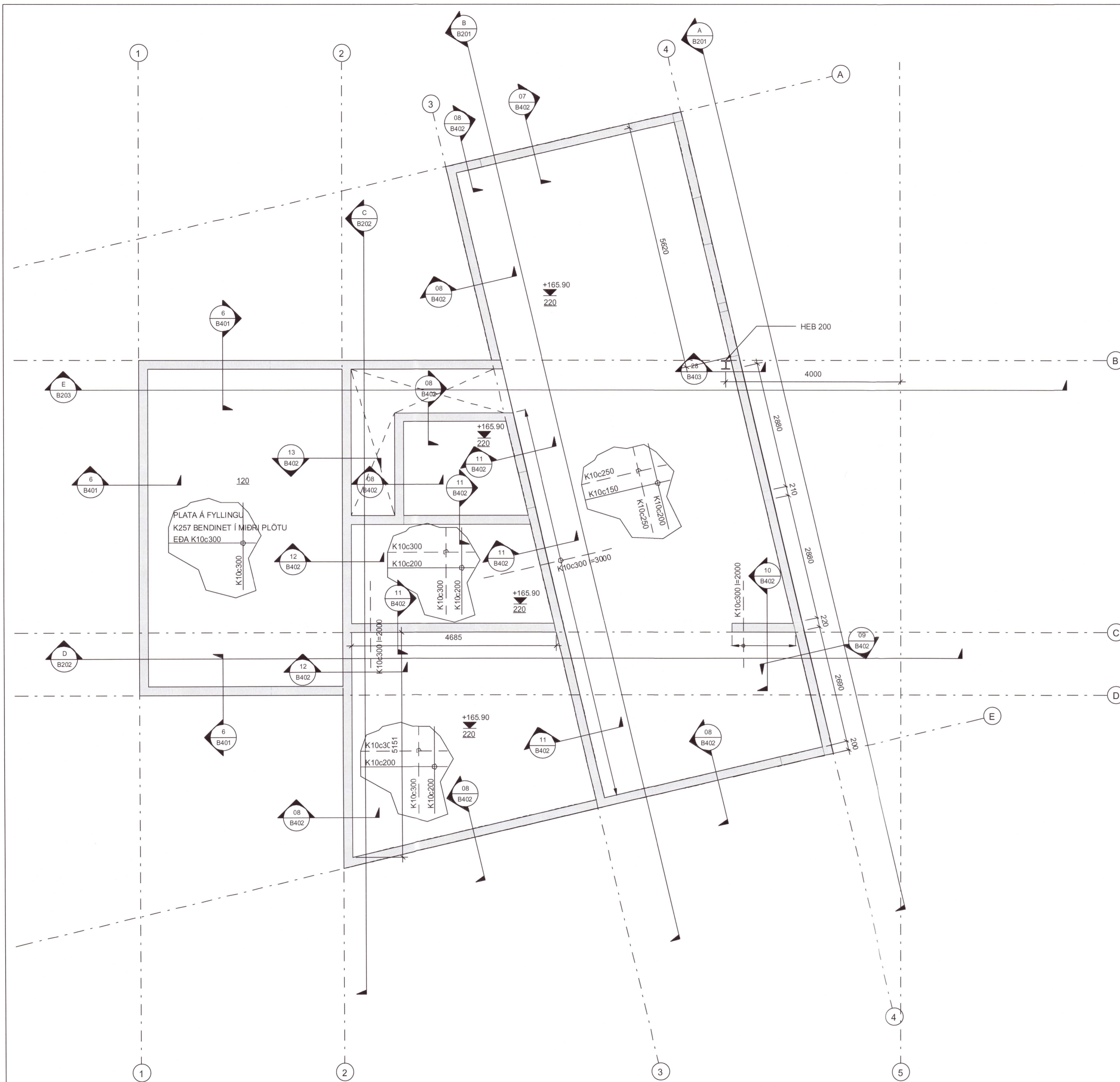
1. Hæð Gólfplata Grunnmynd 1 : 50
