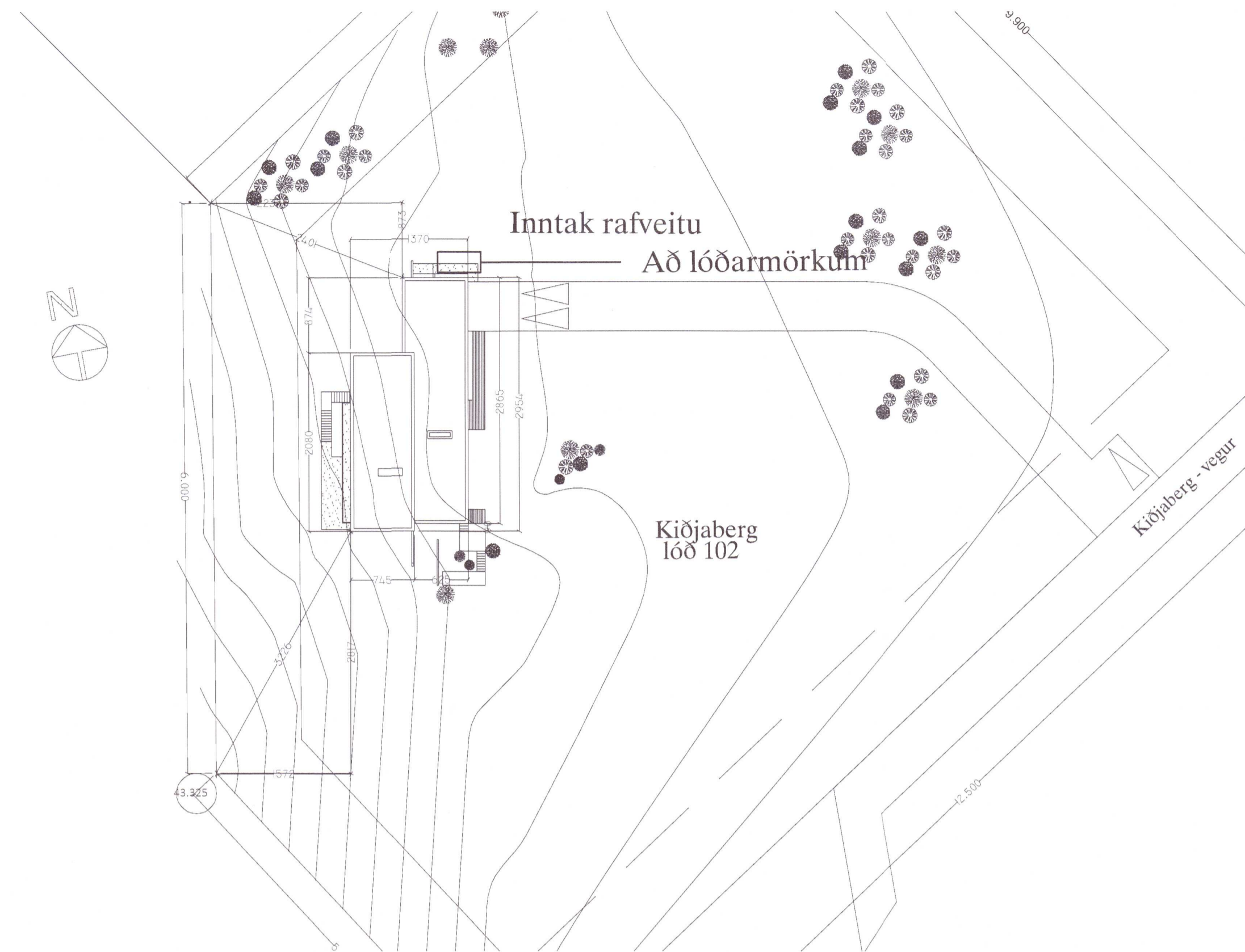
AFSTÖÐUMYND M. 1:500
