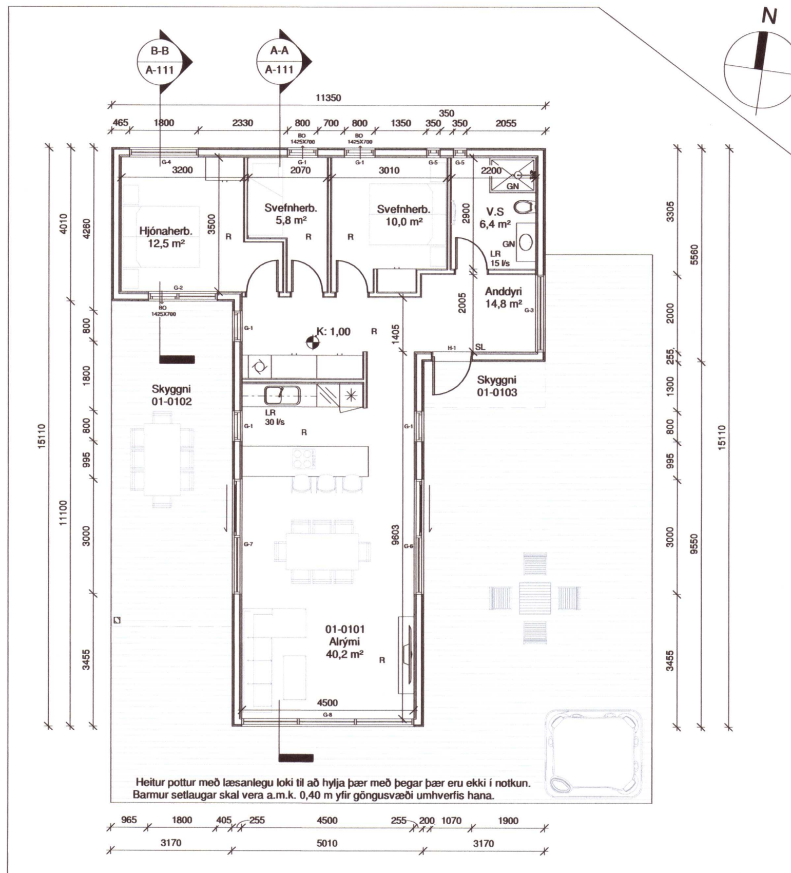
Grunnmynd 1 : 100
