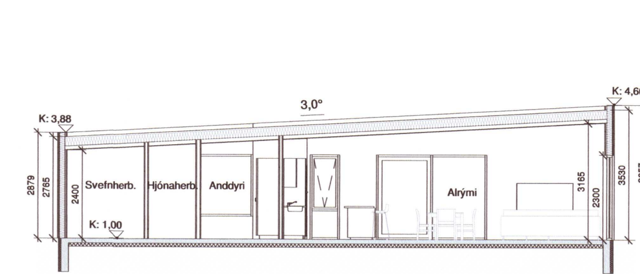
Snið A-A 1 : 100
