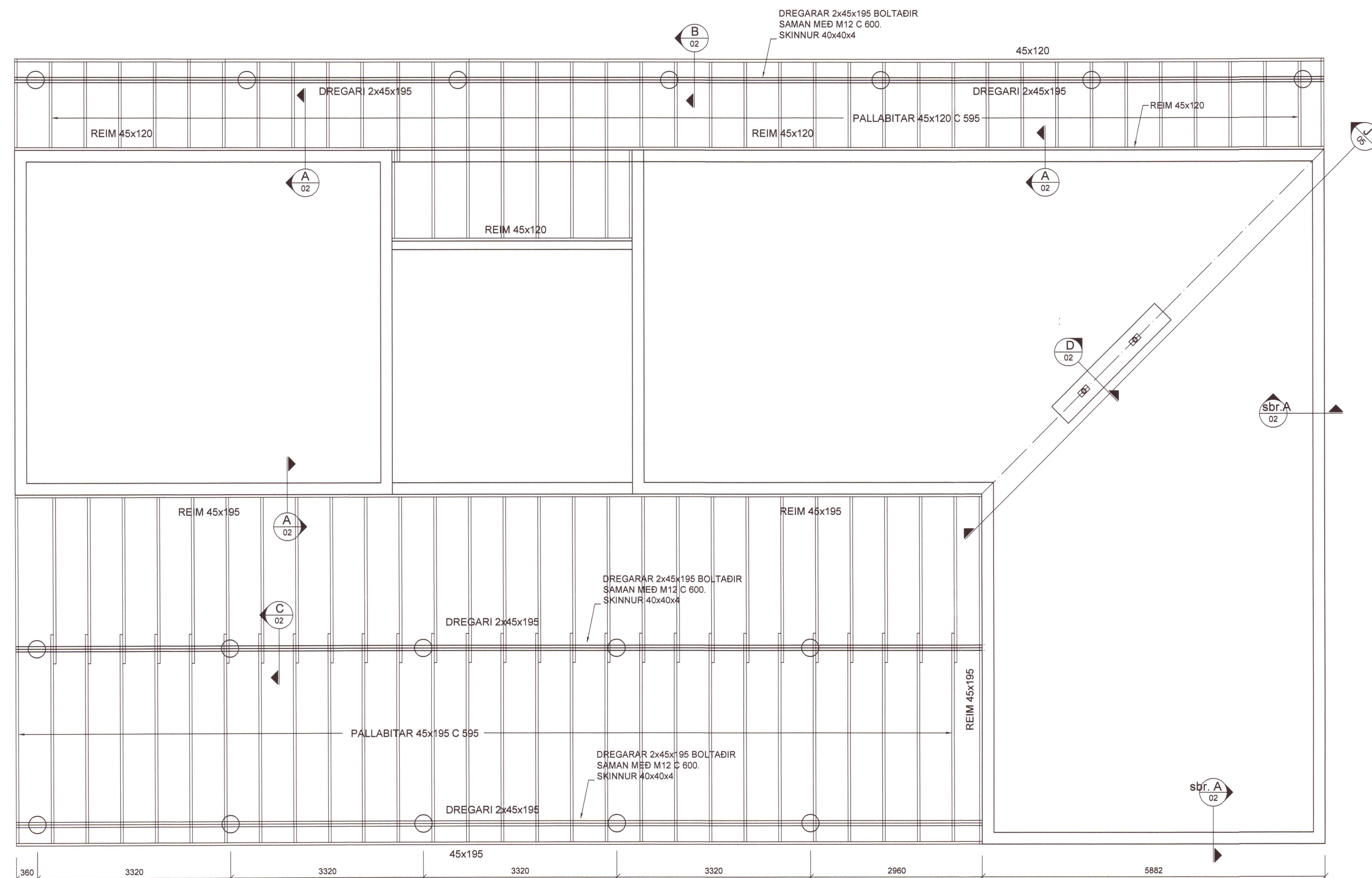
GRUNNMYND PALLUR 1:50
