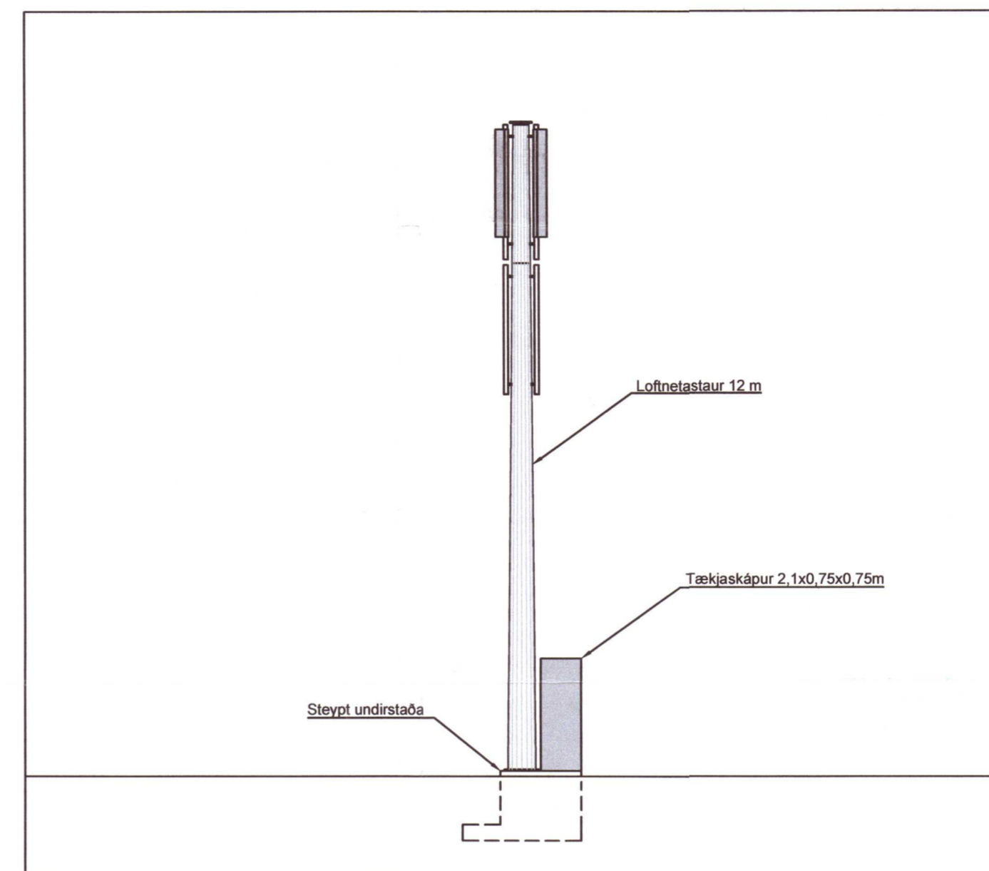
2 Útlit 02 M=1:100
