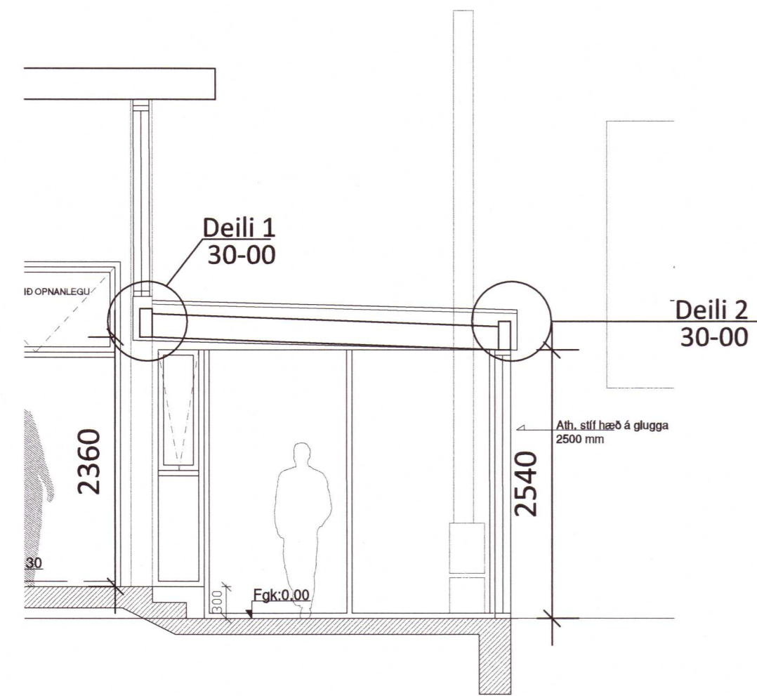
Snið A-A
