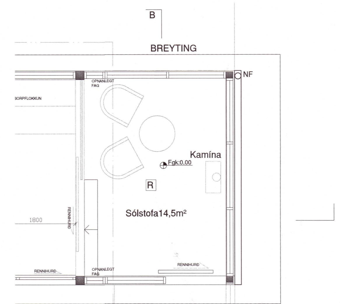
Grunnmynd M. 1:50
