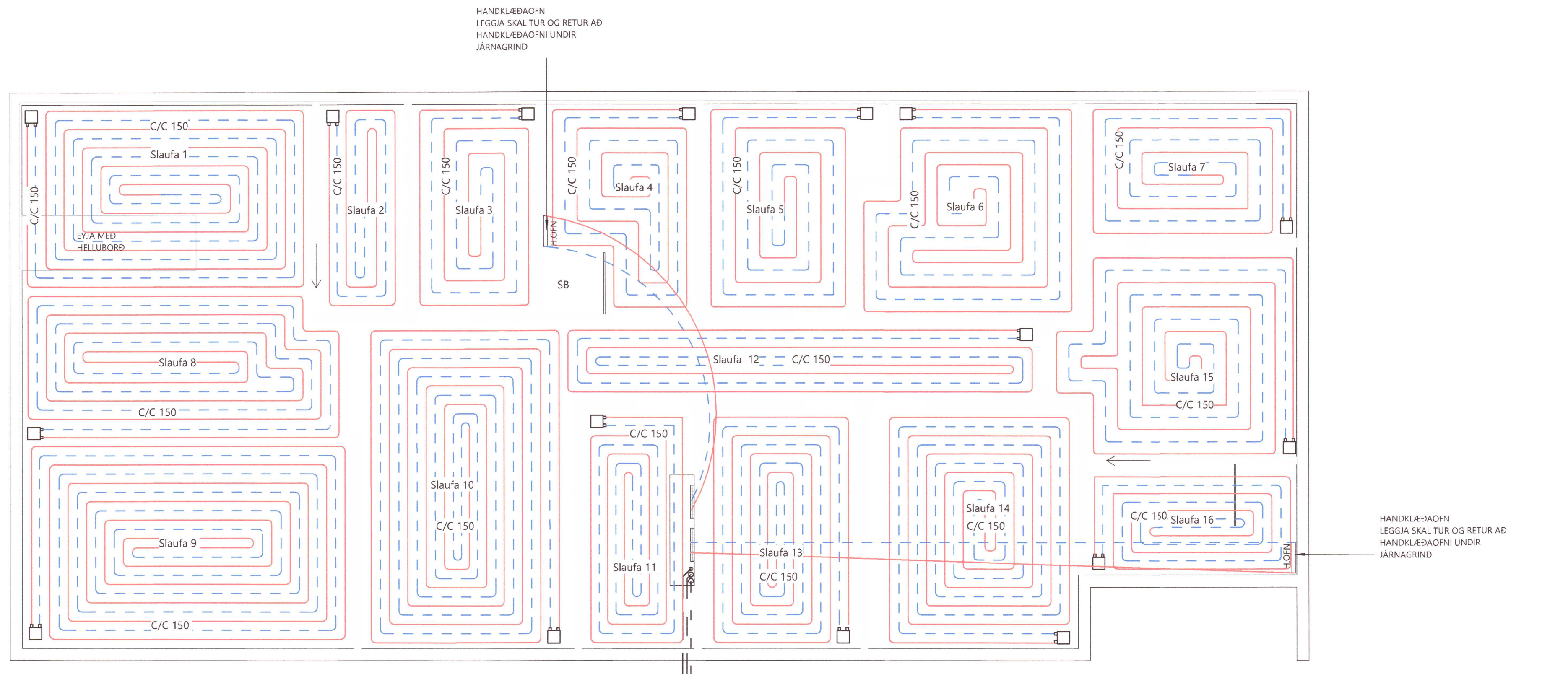
GRUNNMYND GÓLFHITI 1 : 50
