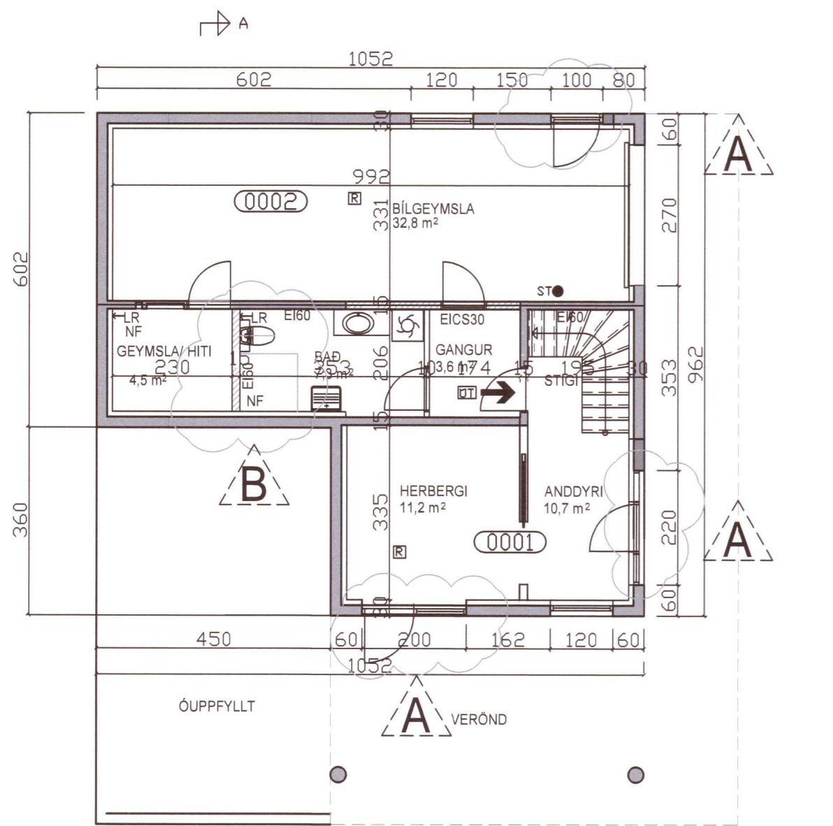
GRUNNMYND NEDRI HÆÐ 1:100
