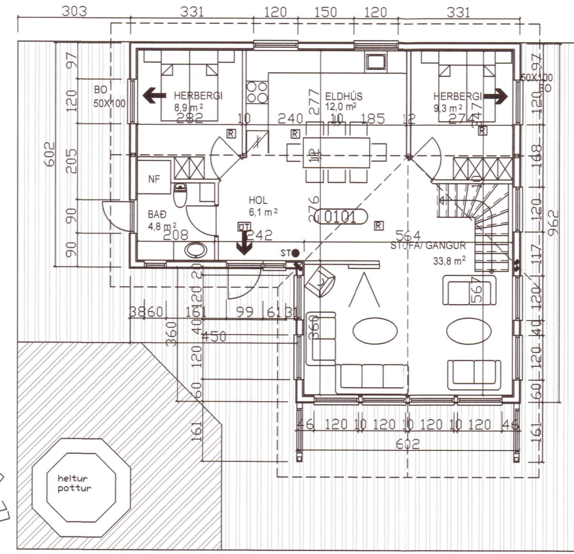
GRUNNMYND EFRI HÆÐ 1:100
