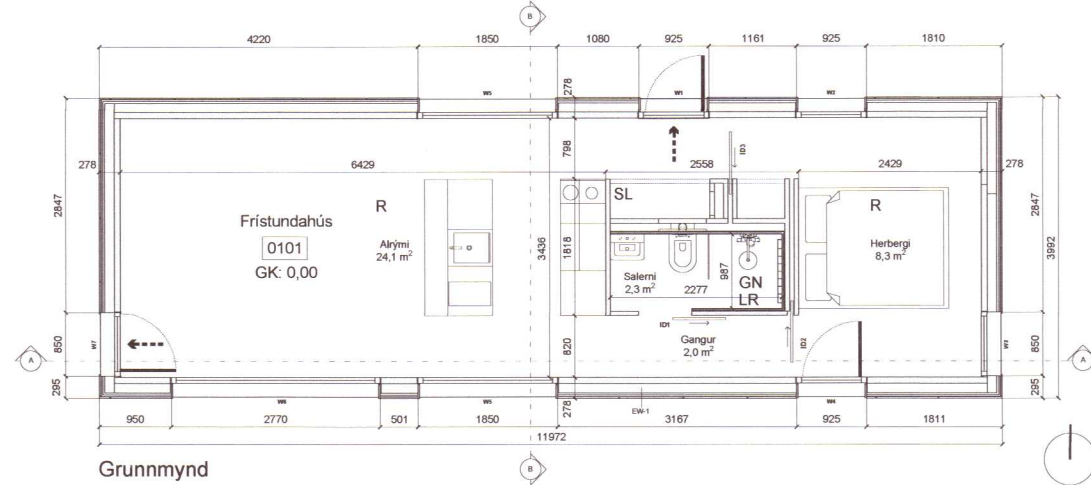
Grunnmynd
