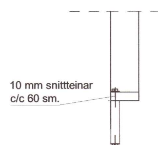
Festing fótreim við gólfbita 1 : 20
