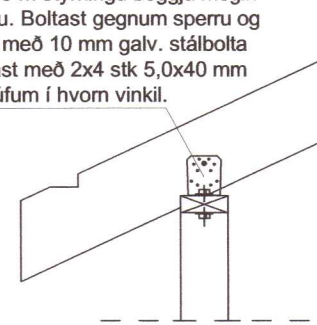
Festing sperru við vegg deili 1 : 20
