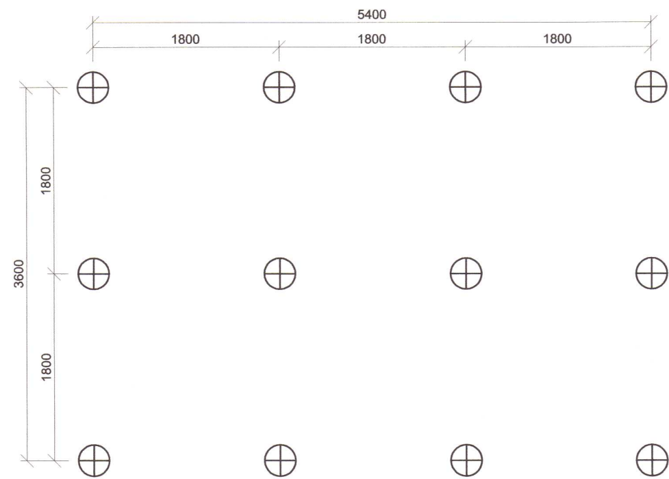
UNDIRSTÖÐUR
