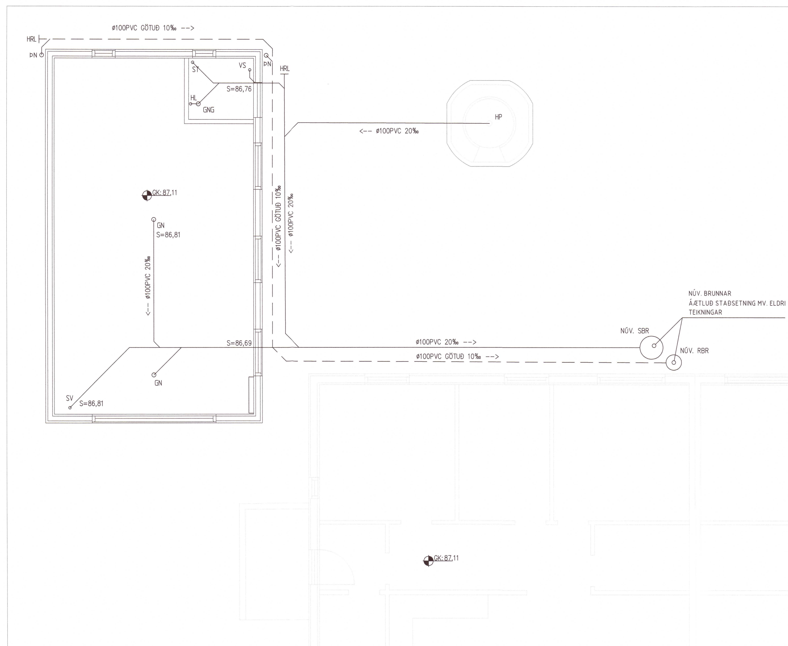
GRUNNMYND 1:50
