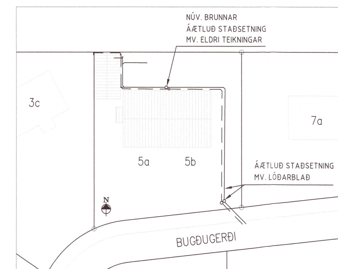
AFSTÖÐUMYND 1:500
