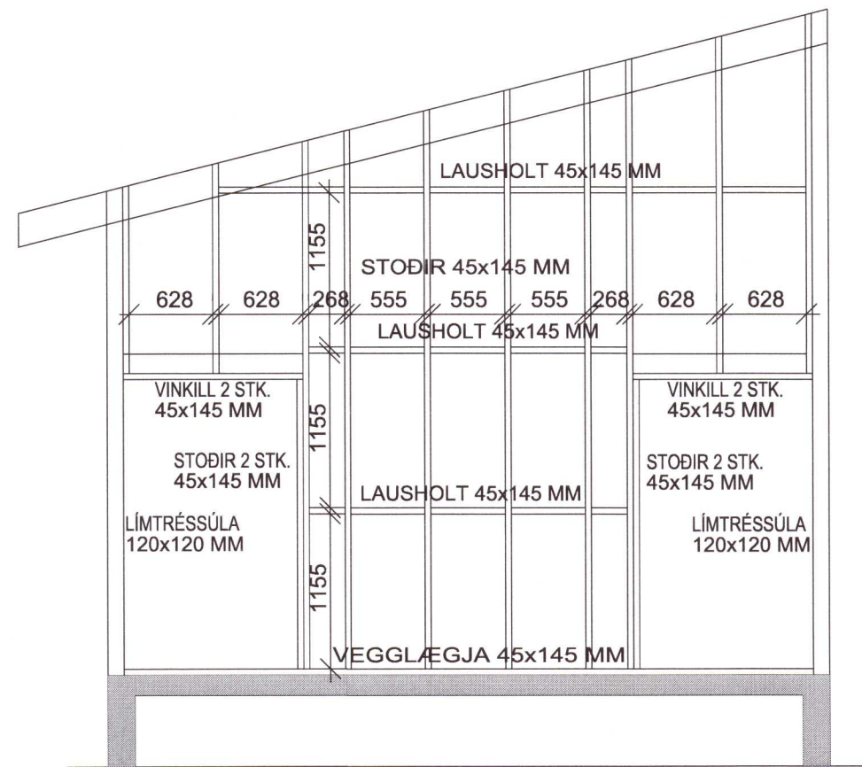
SNID - E 1:50
