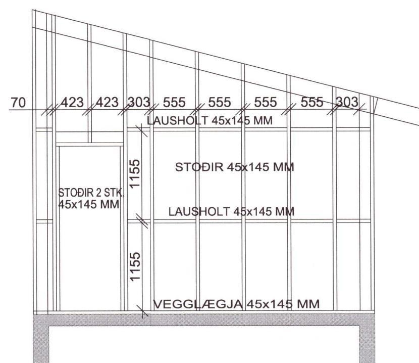
SNID - G 1:50
