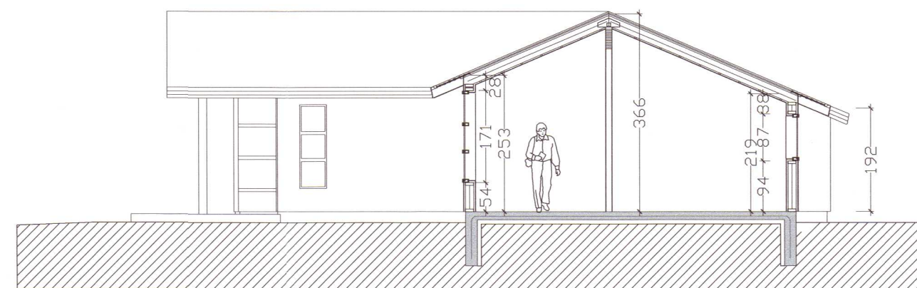
Snið B-B
