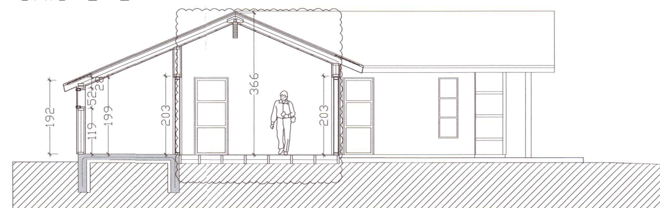
Snið C-C
