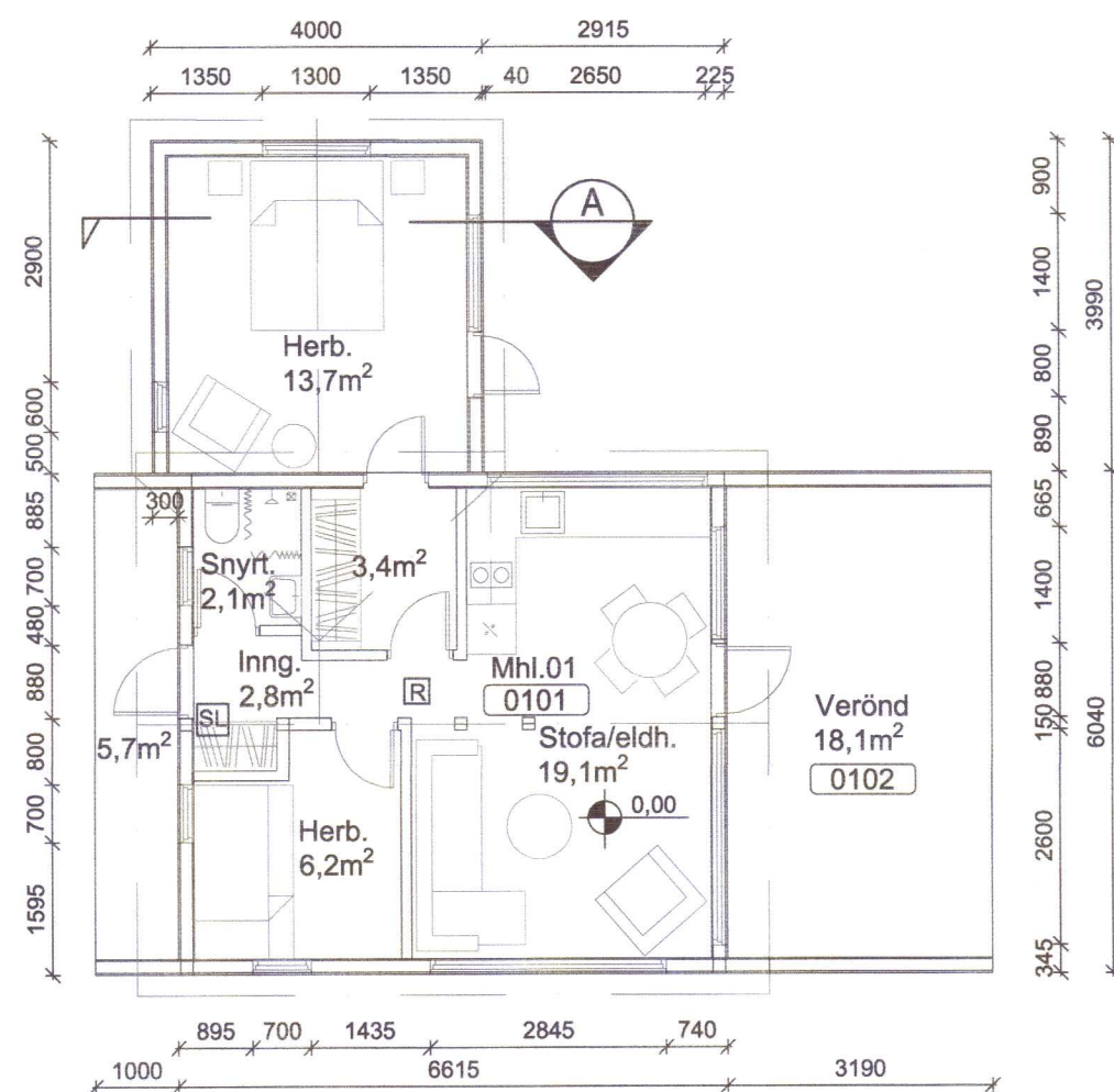
Grunnmynd M 1:100
