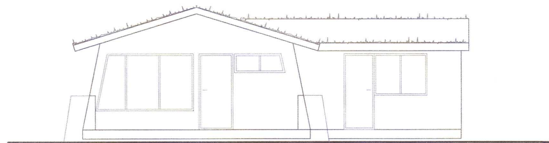
Suðurhlíð M 1:100
