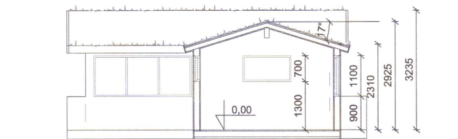
Sneiðing M 1:100
