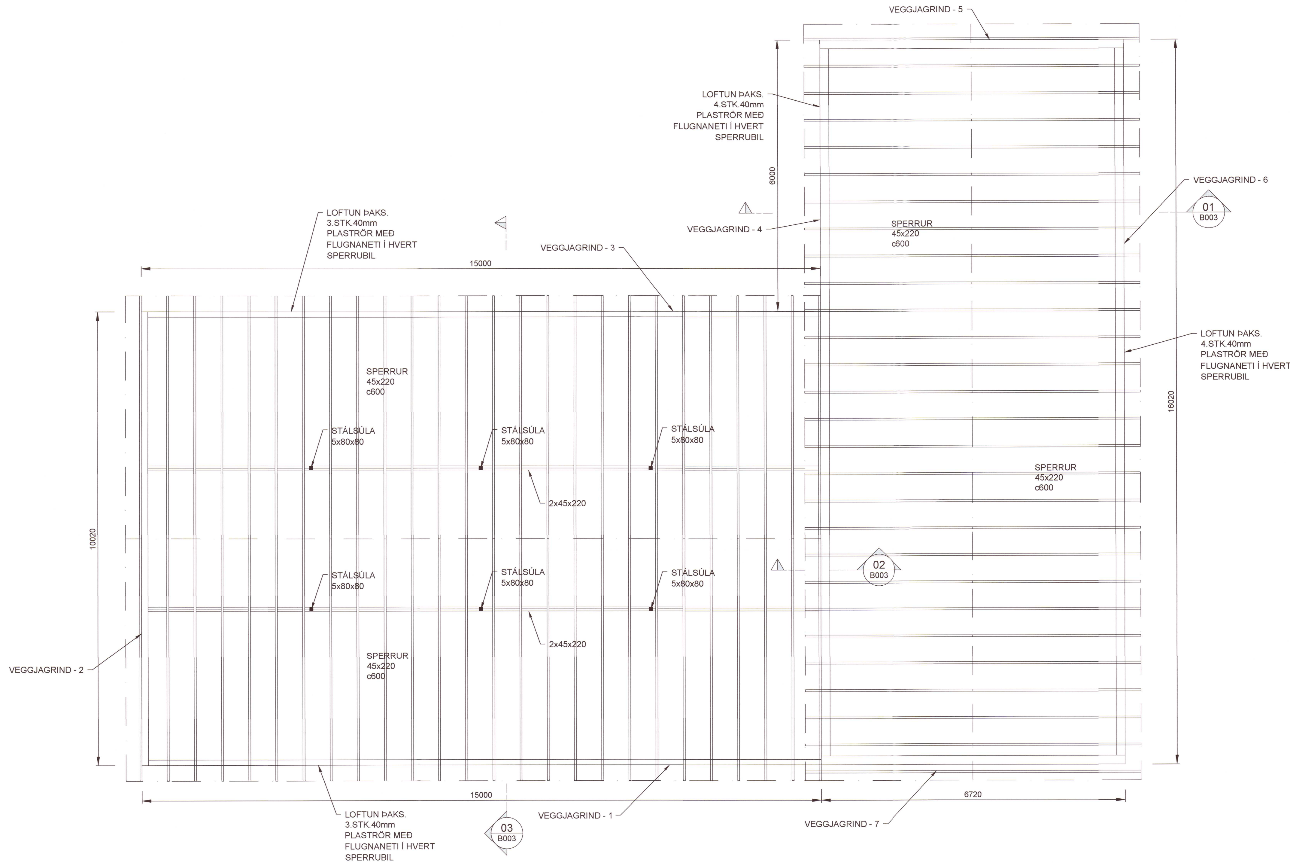
GRUNNMYND - ÞAKVIRKI 1:50 (A1)
