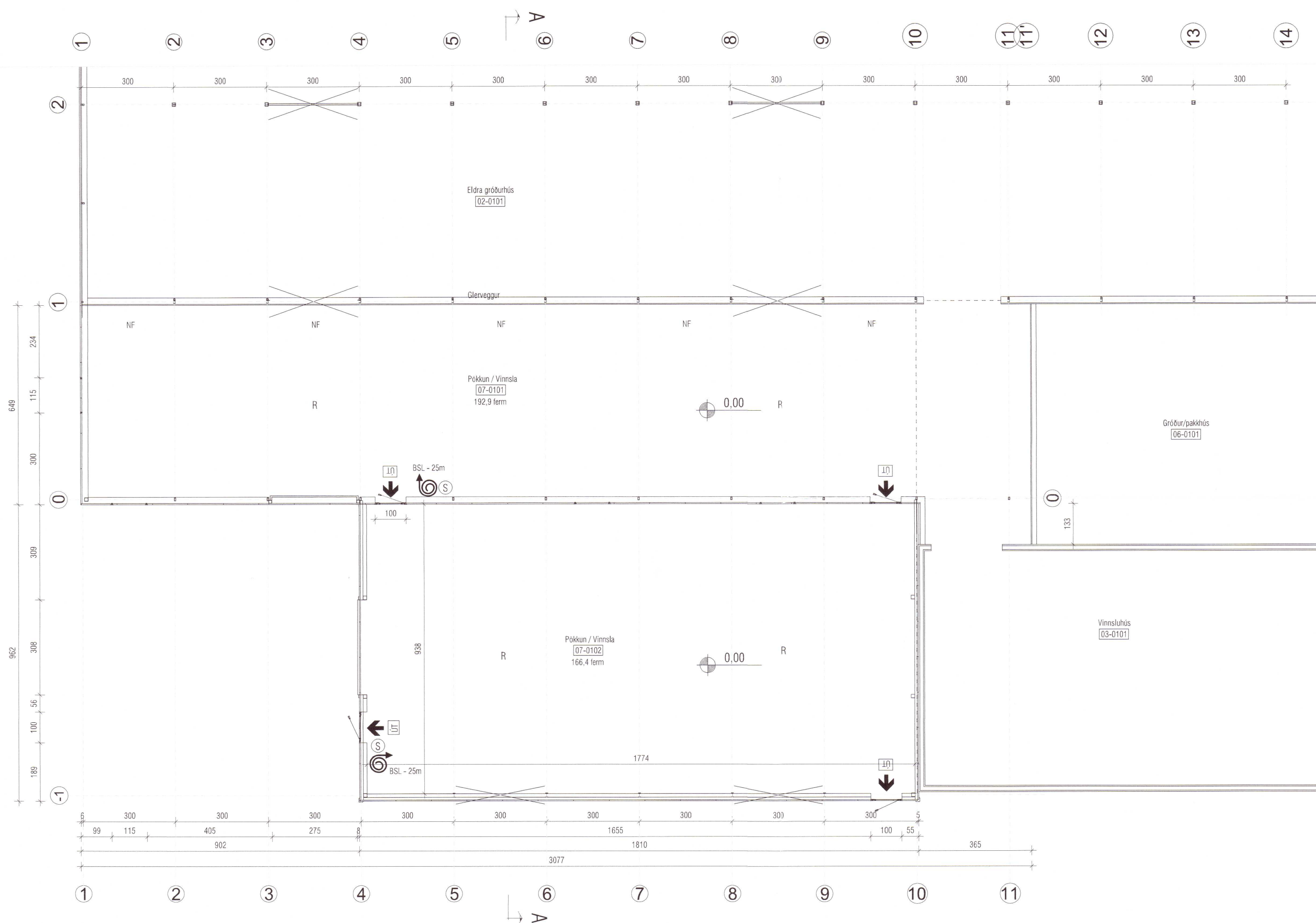
GRUNNMYND - 1:100
