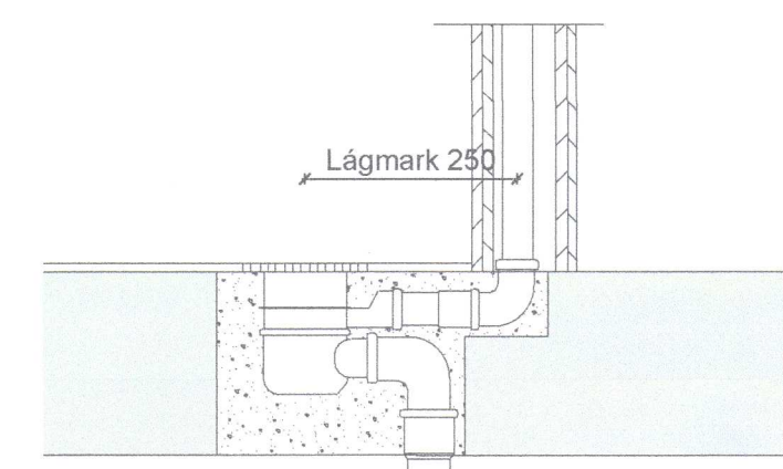
GÓLFNIÐURFALL MEÐ GEGNUMRENNSLI, MKV...1:10
