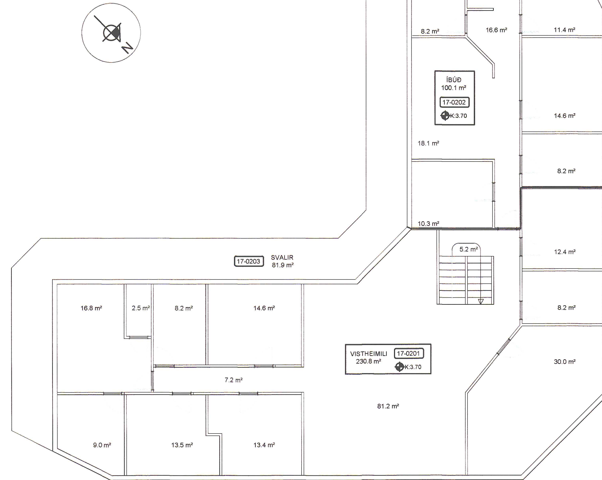
GRUNNMYND EFRI-HÆÐAR Mkv. 1:100
