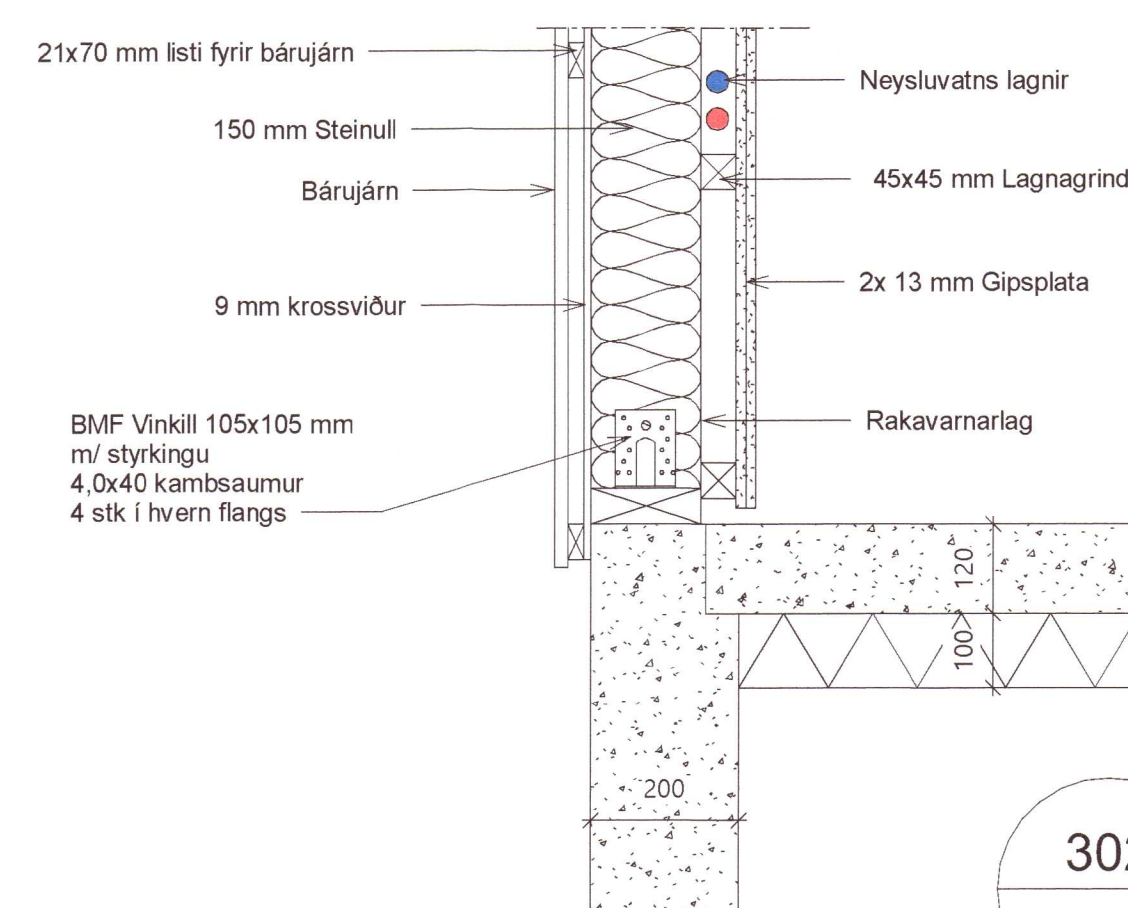
L 03 Neysluvatnslagnir í útvegg 1 : 10
