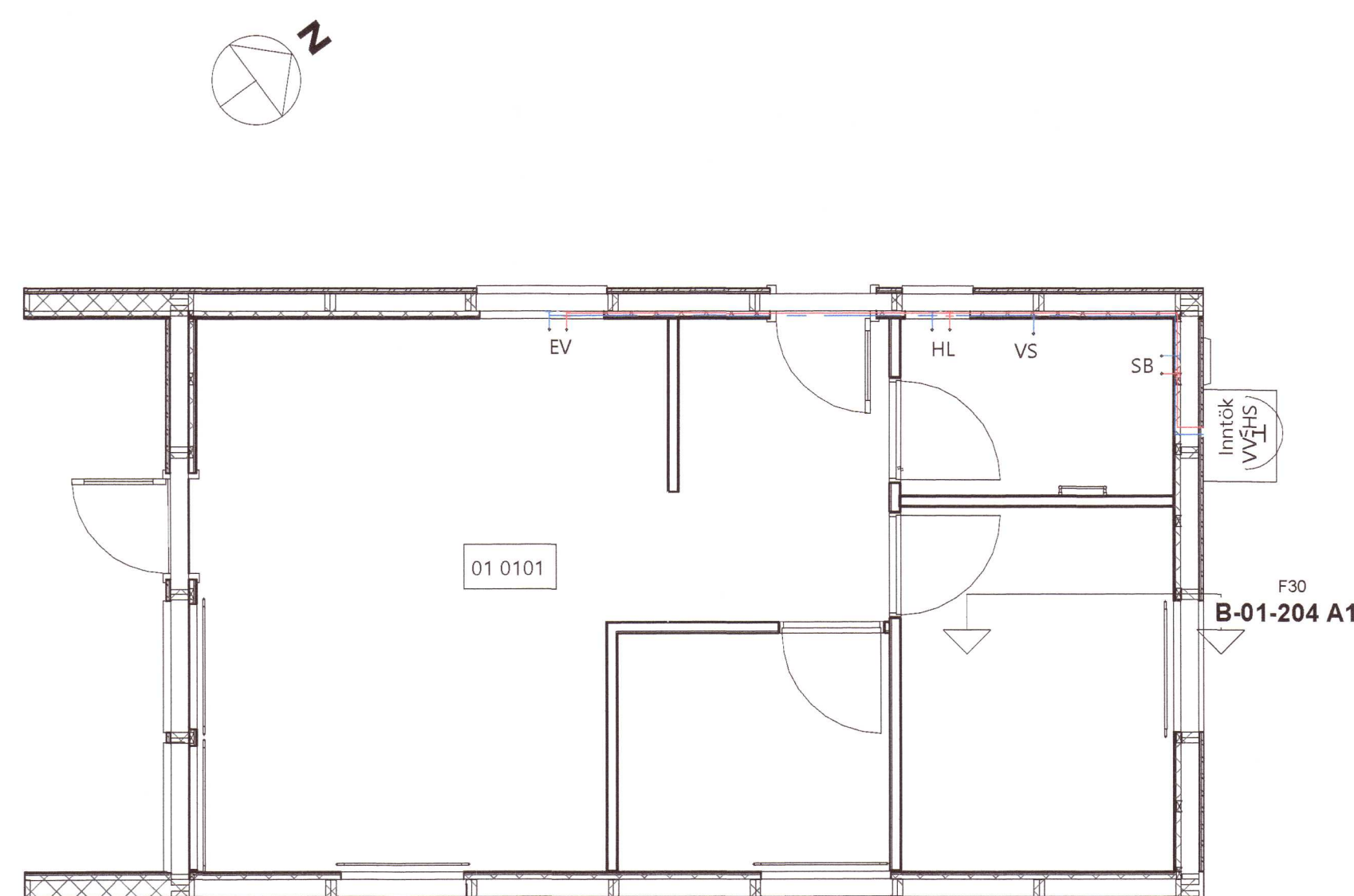
01 Grunnmynd Neysluvatnslagnir 1 : 50
