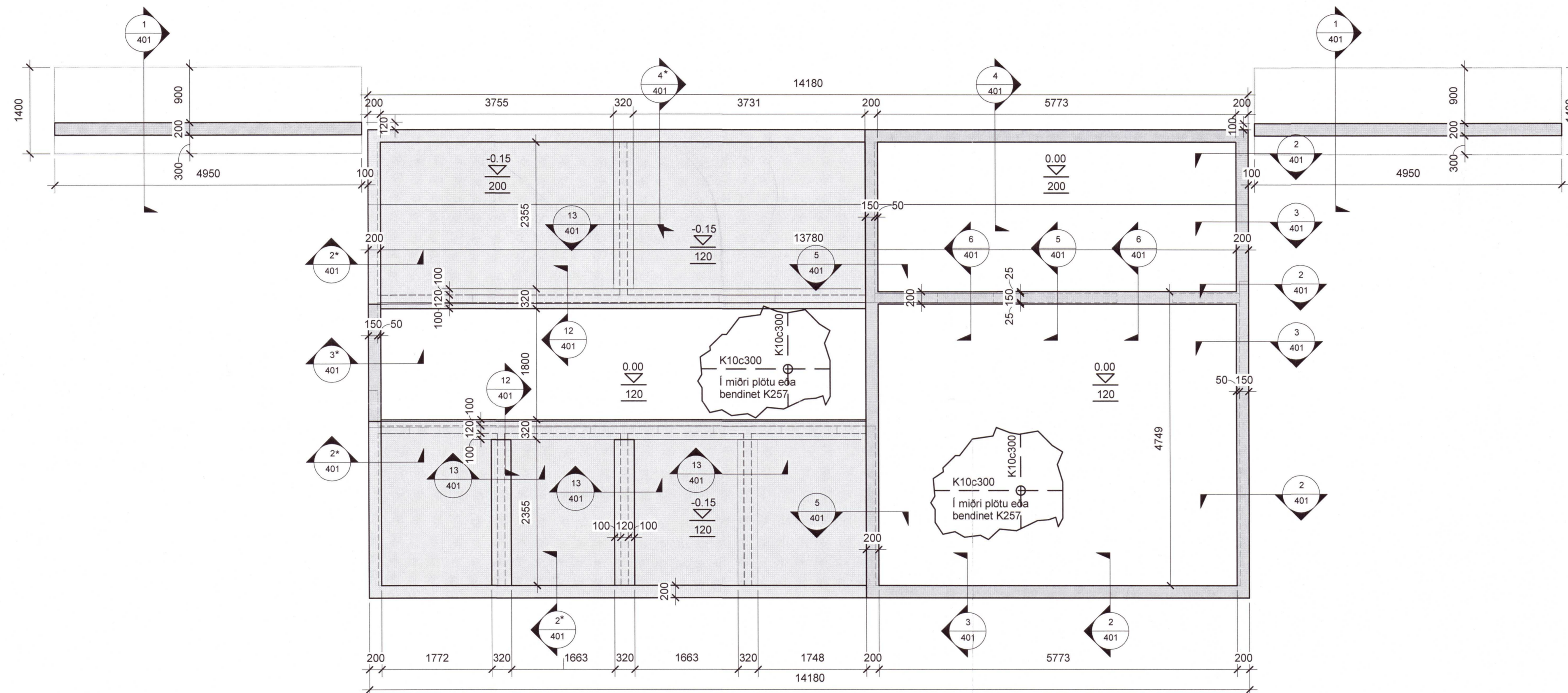
1 00 sökkjar - Hesthús 1 : 50
