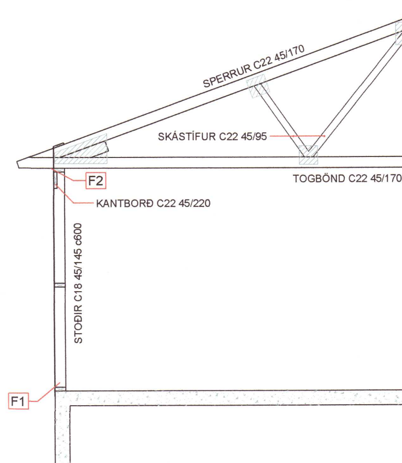
SNIÐ B1 Mkv. 1:50
