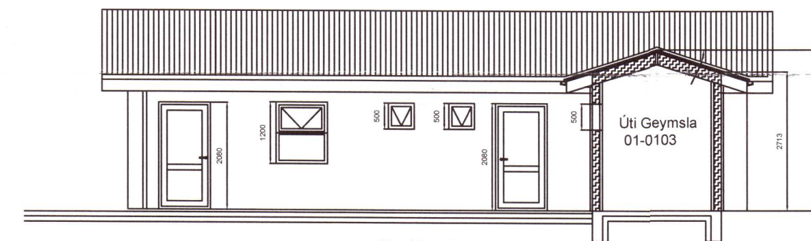
Snið B
