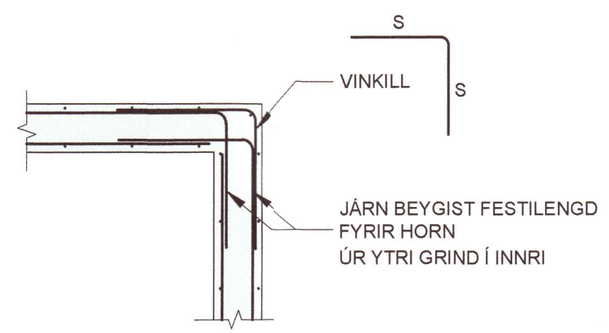
LÁRETT SNIÐ Í VEGGHORN Mkv 1:20
