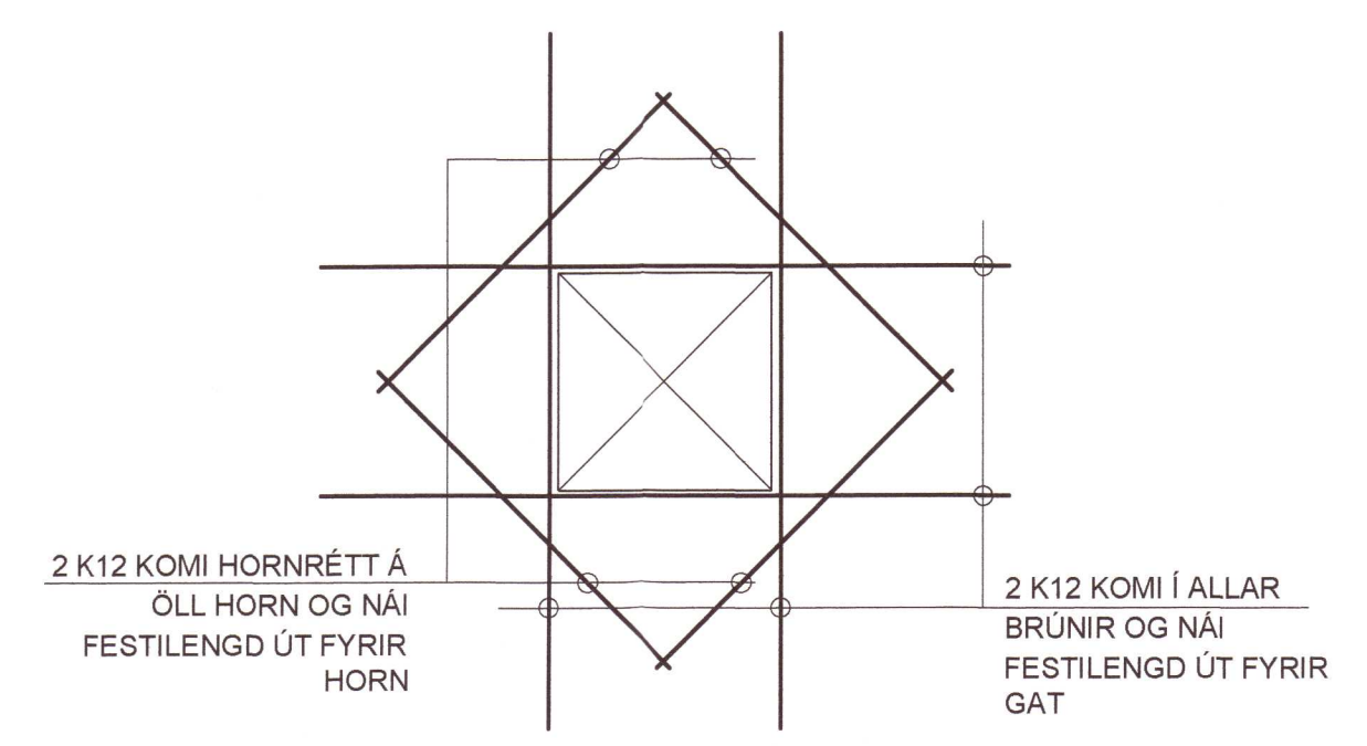
BENDING Í KRING UM ÖP Mkv 1:20
