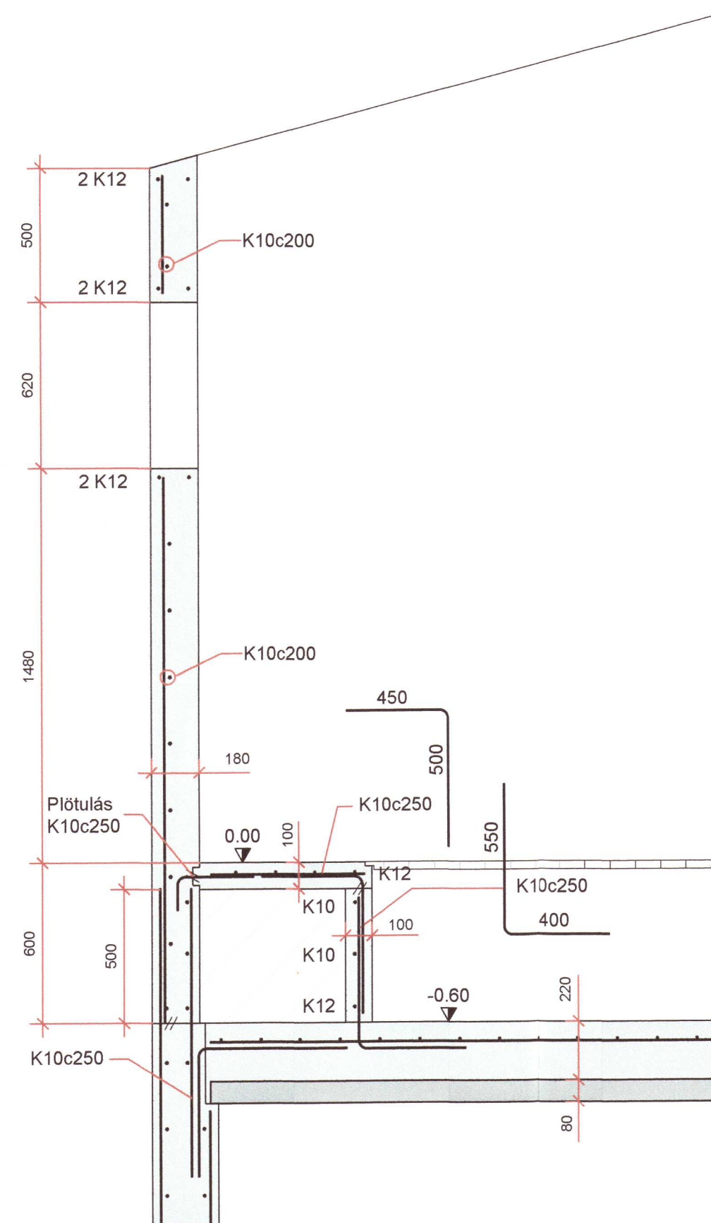
C SNIÐ B02 Mkv. 1:20
