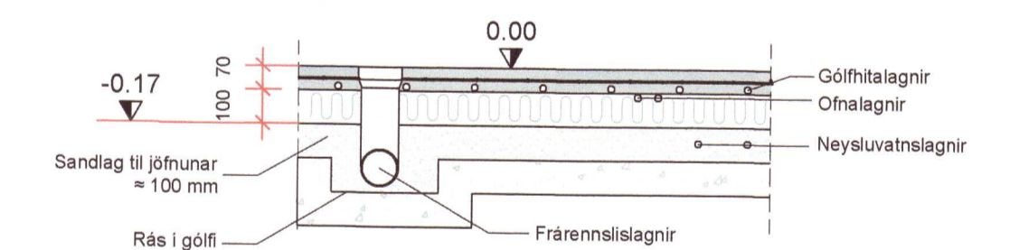
ALMENNT SNIÐ Mkv. 1:20
