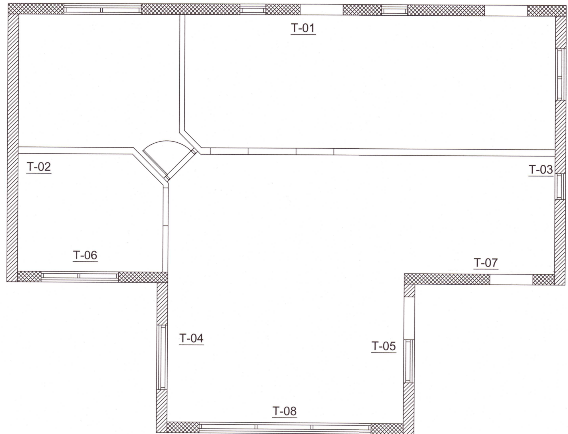
GRUNNMYND 1:50
