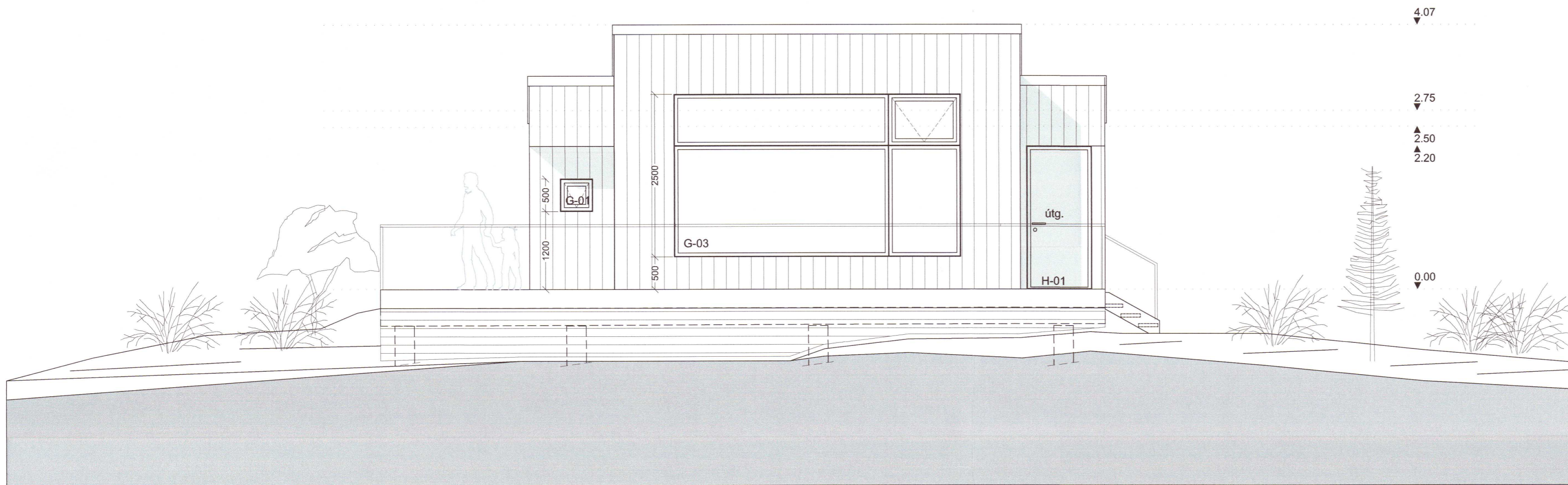
Útlit til suðausturs 1:50
