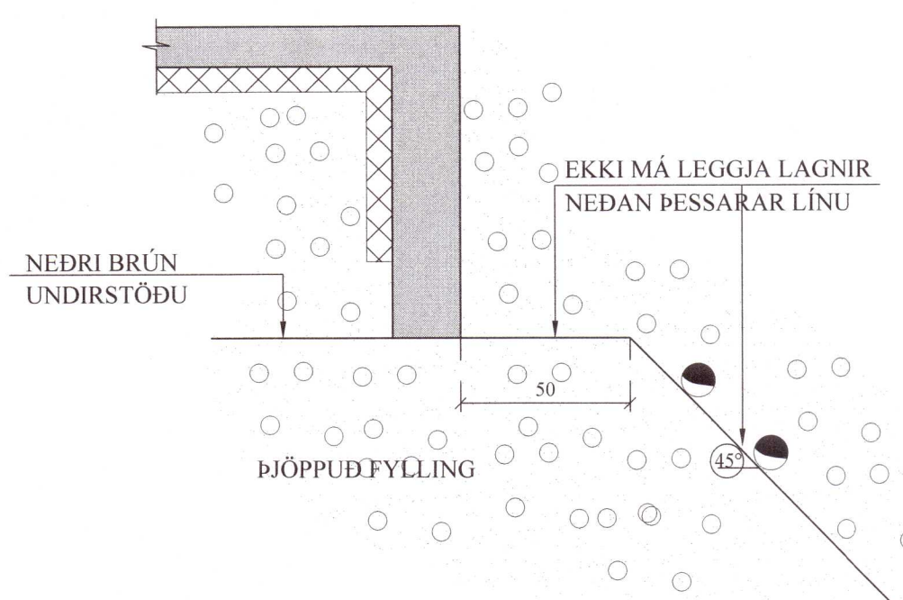
LEGA LAGNA VIÐ UNDIRSTÖÐUR. 1:20
