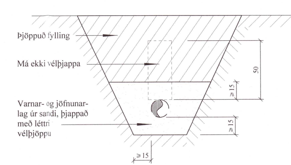
FRÁRENNSLISLAGNIR Í JÖRÐU OG GRUNNI. 1:20
