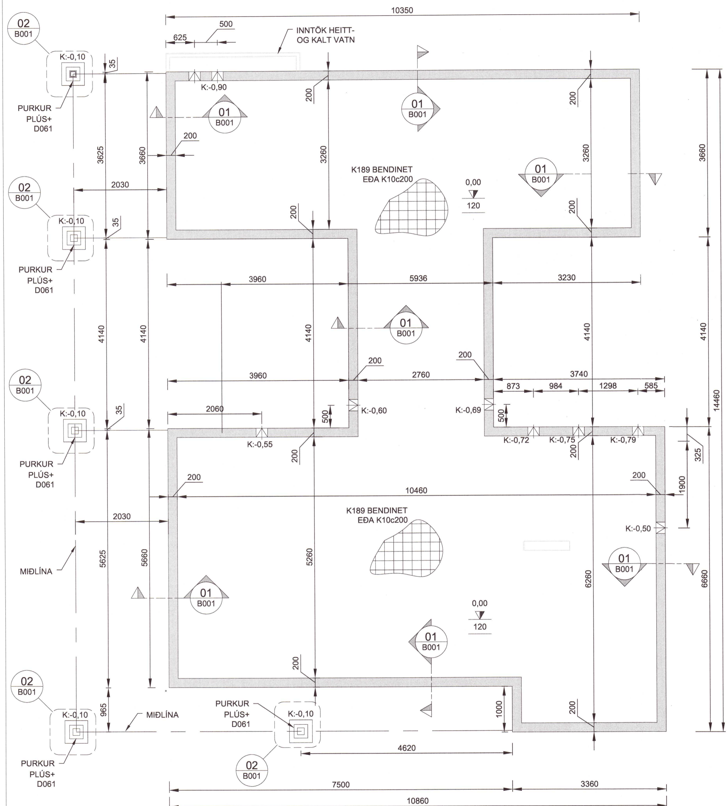
GRUNNMYND - UNDIRSTÖÐUR 1:50 (A2)
