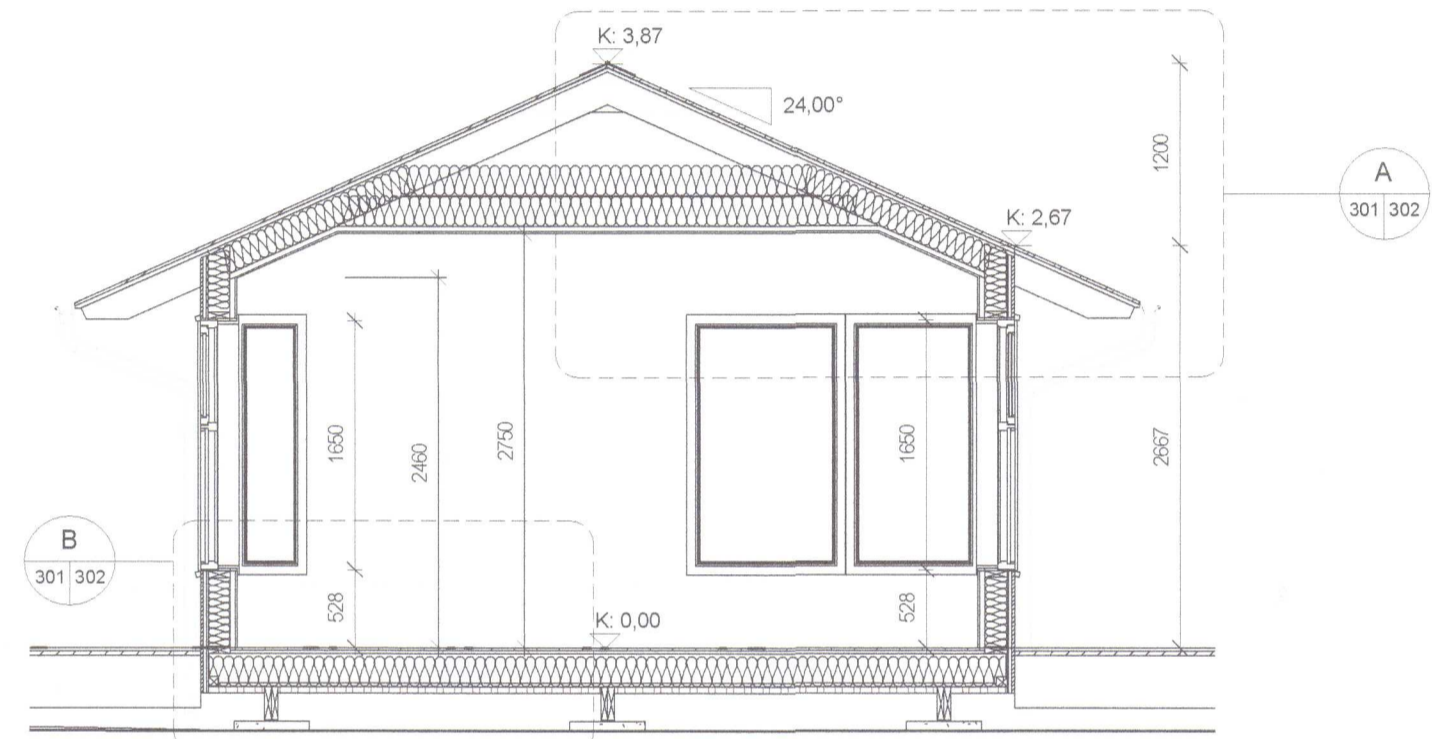
Snið A. 1 : 50
