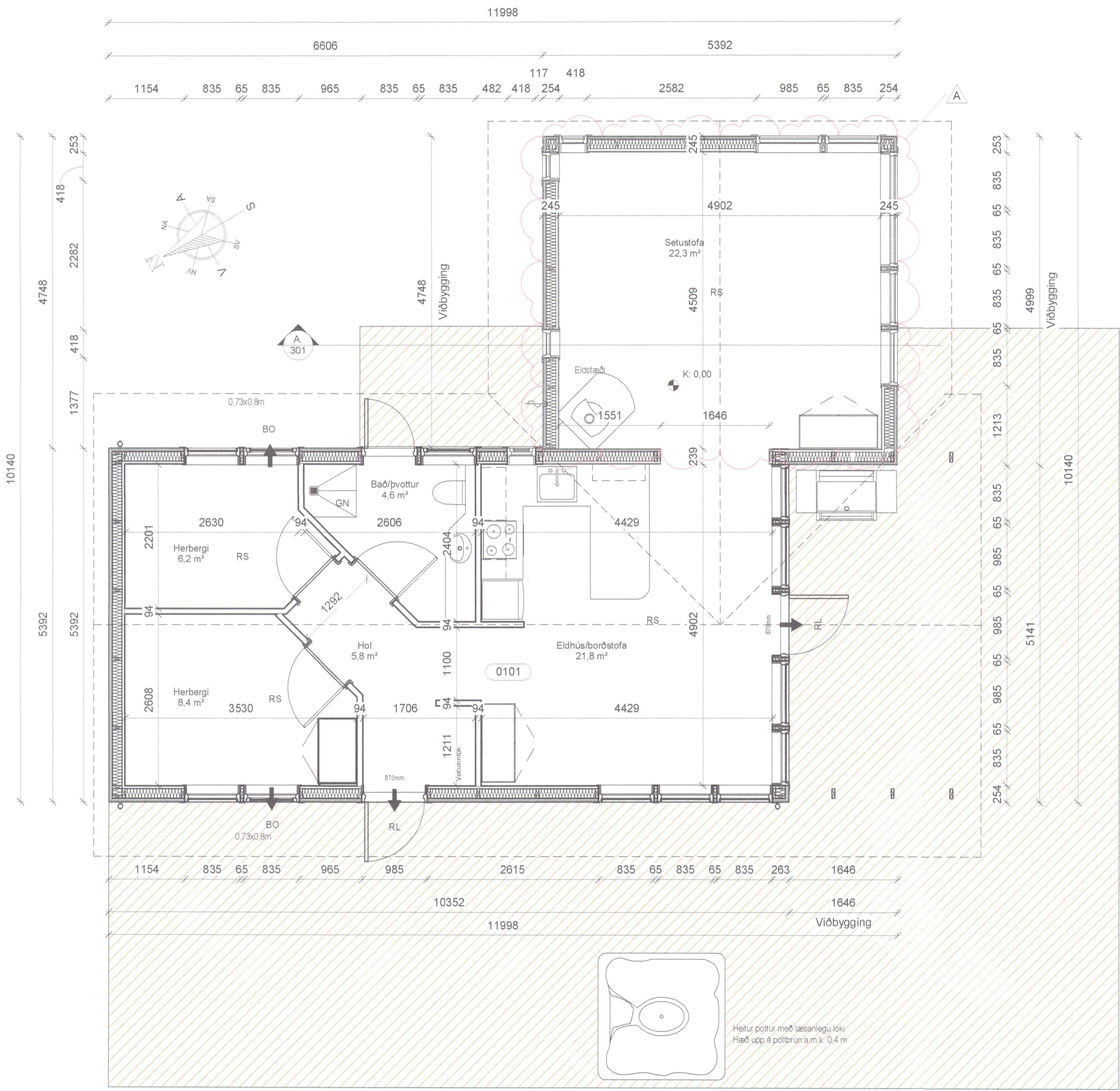
Grunnmynd 1 : 50
