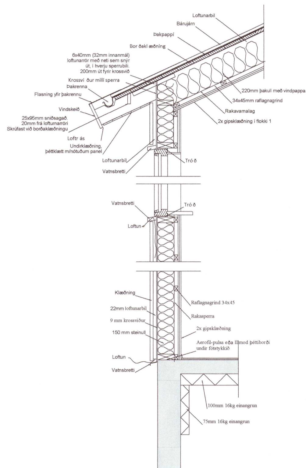
Lóðrétt sneið í útvegg mkv. 1:20
