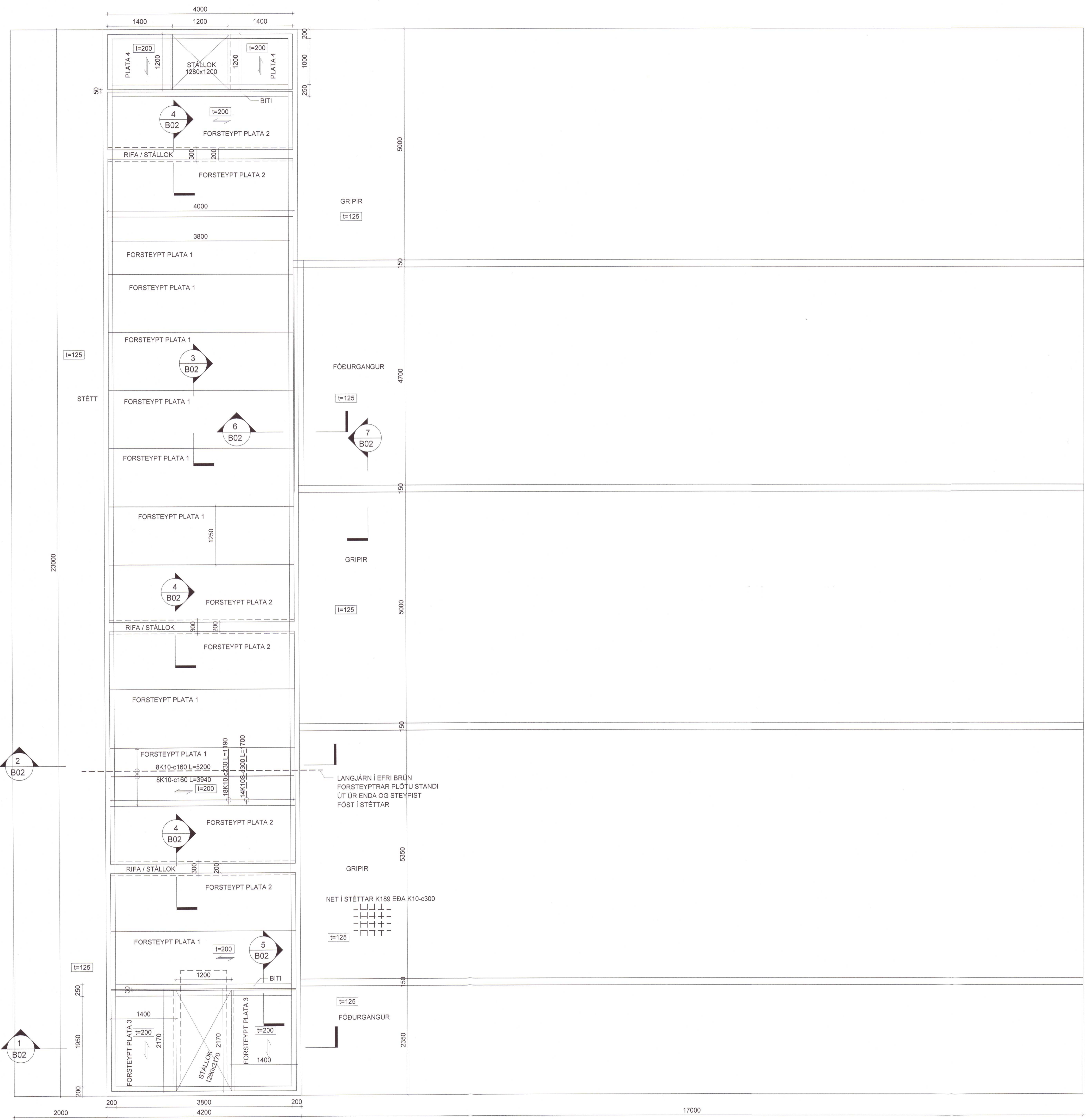
2 Grunmynd haugkjallara og stétta 1 : 50
