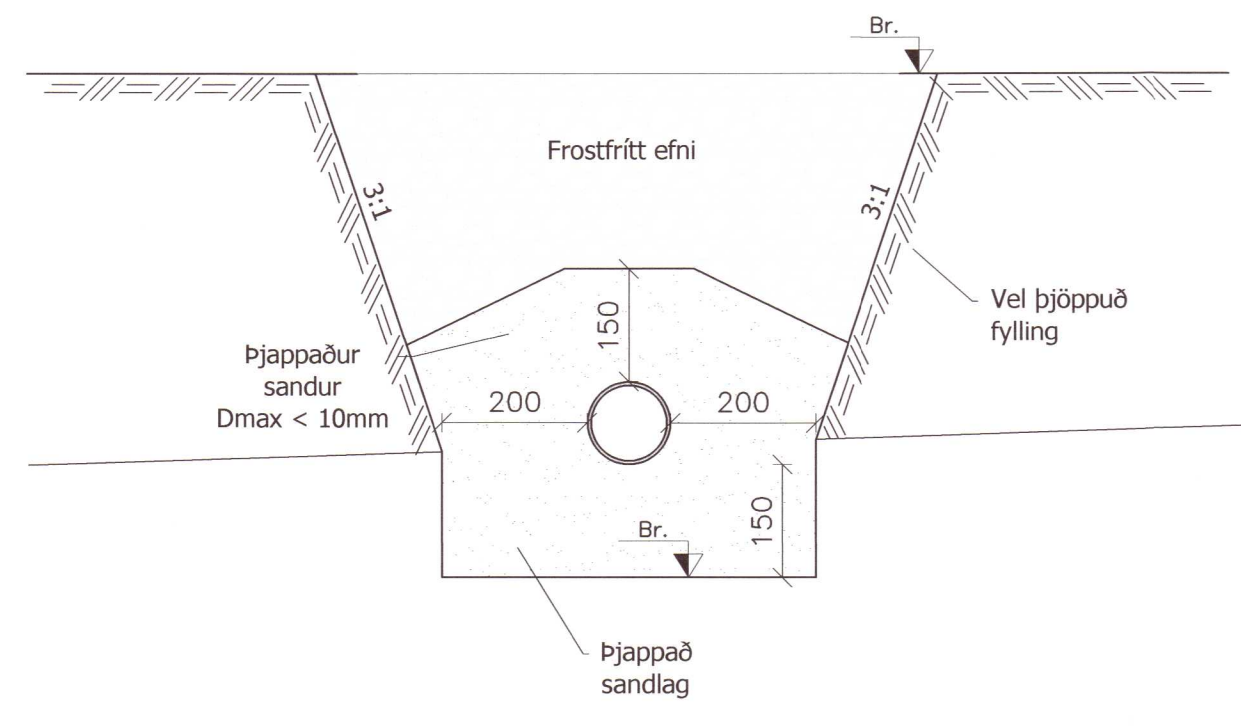
A Snið – Fráveitulagnir, almennt skurðsnið Mkv: 1:10
