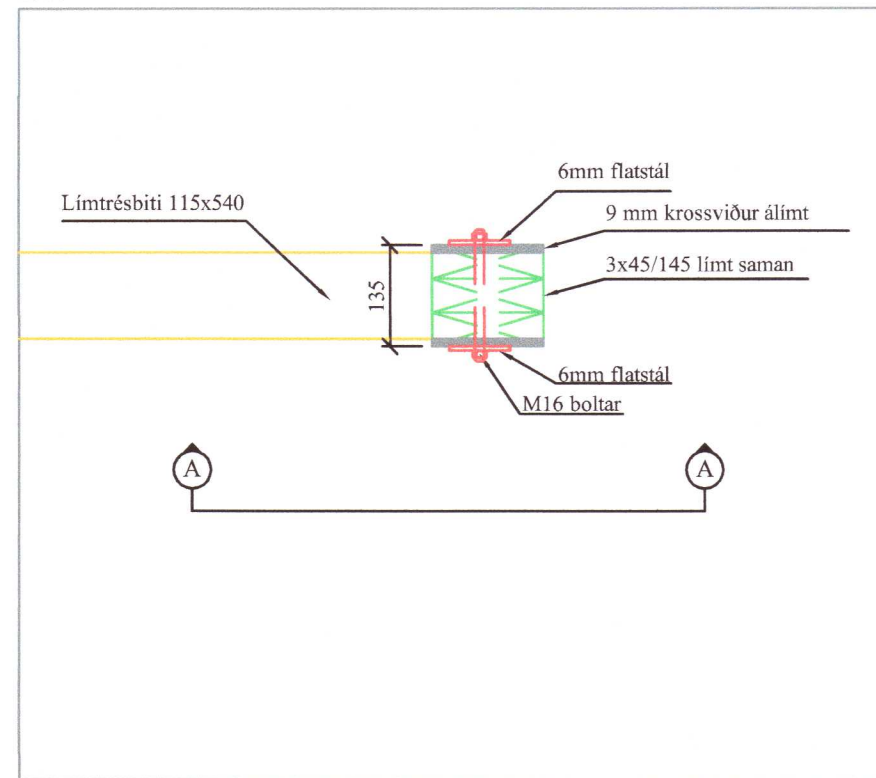
S3-Grunnmynd 1:10
