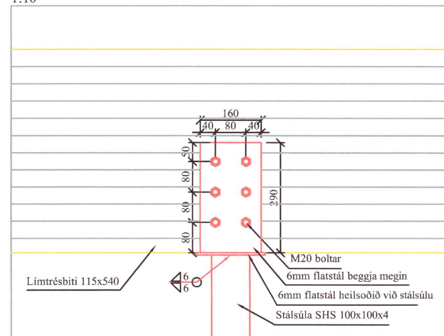
S2-Ásýnd/grunnmynd 1:10
