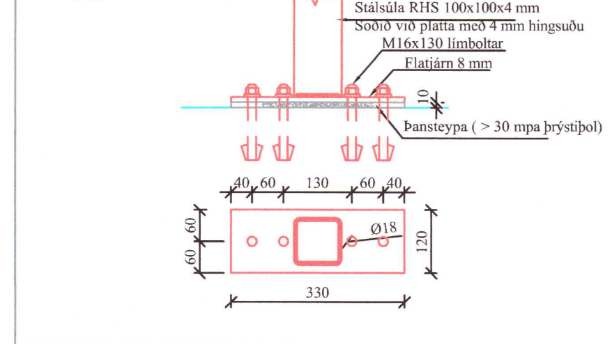
S2-Ásýnd/grunnmynd 1:10
