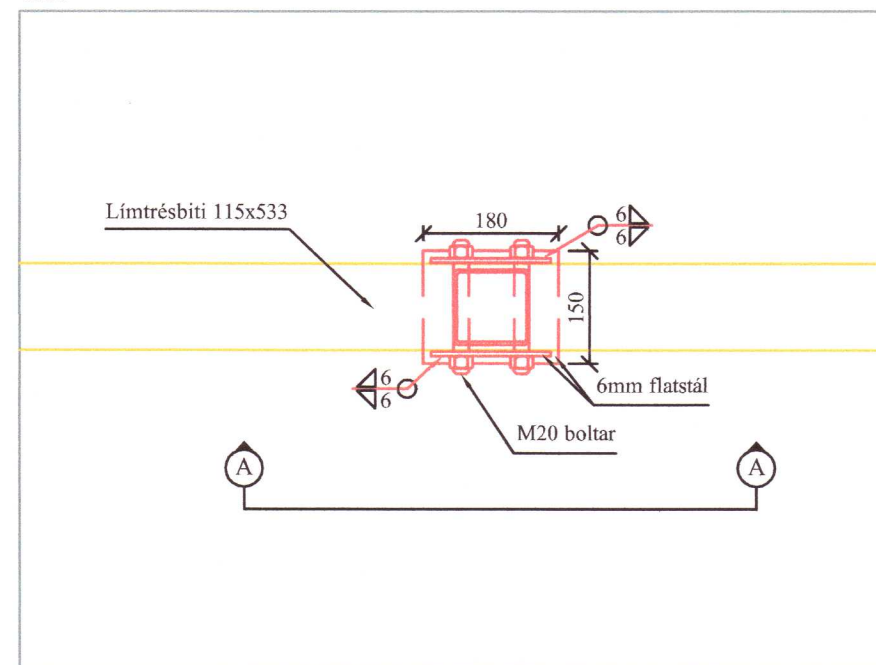
S3-Grunnmynd 1:10
