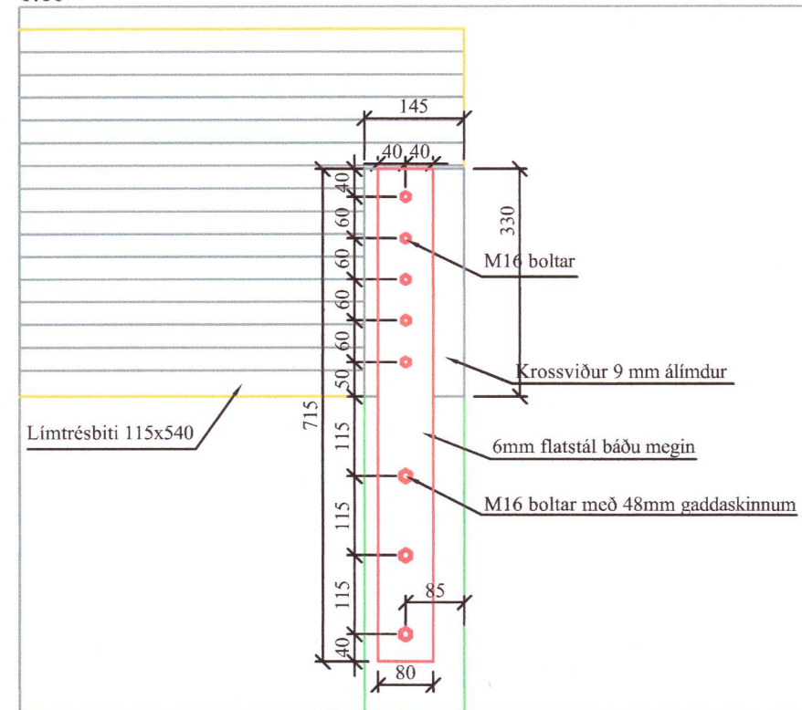
S3-Ásýnd A-A 1:10
