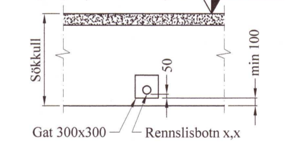
Skýringamynd af inntaksgati GK:
