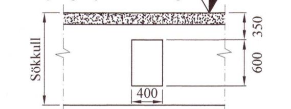
Skýringamynd af inntaksgati GK:
