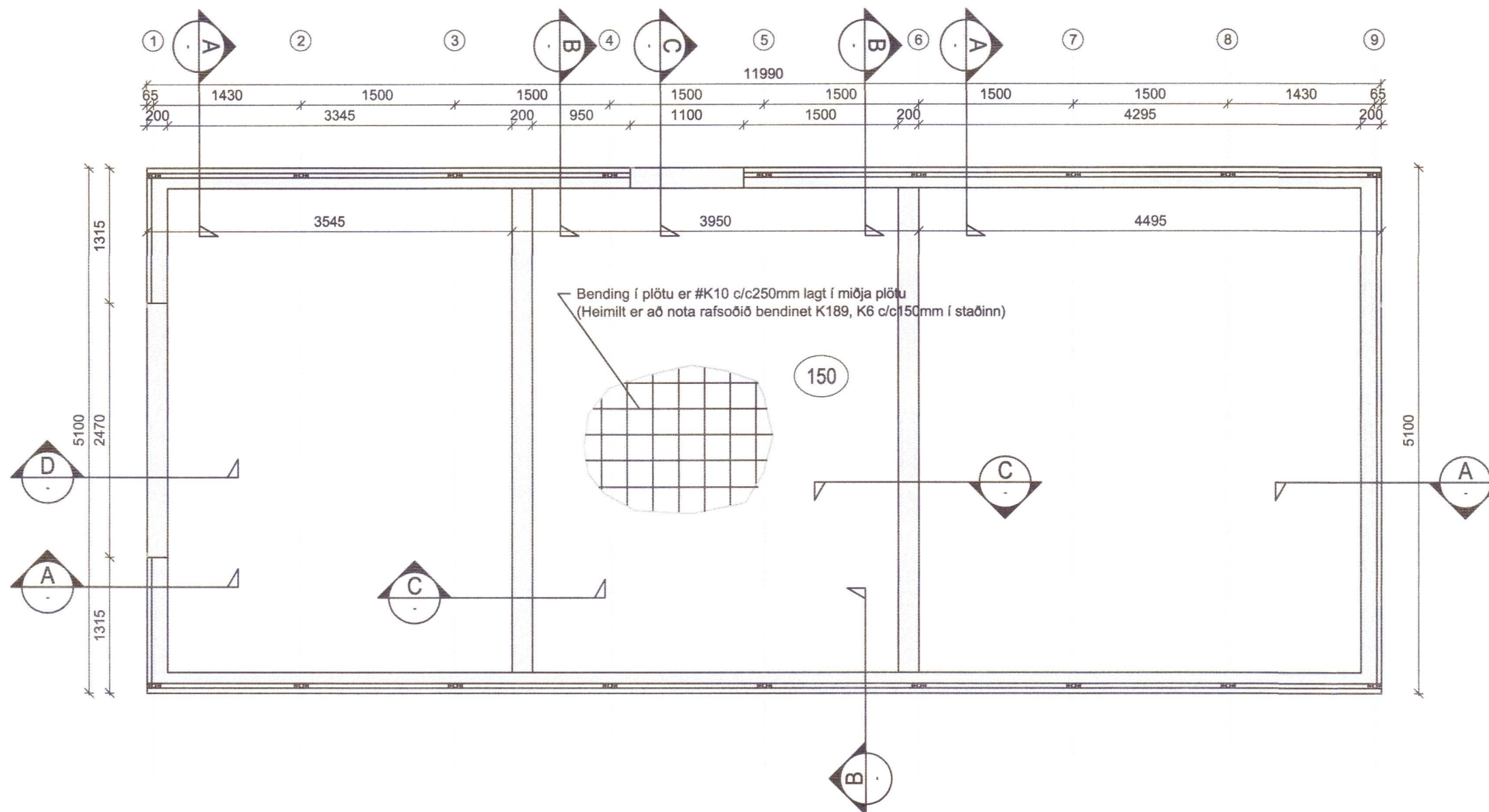
Undirstöður - grunnmynd M 1:50
