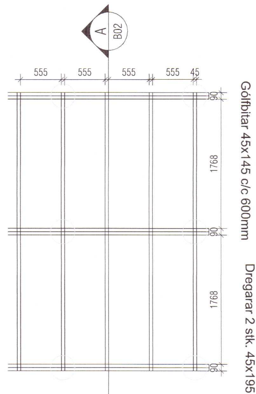
GRUNNMYND GÓLFBITA Mkv. 1:50
