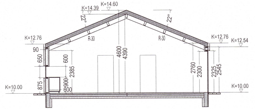
SNEIÐMYND A, MKV. 1:100
