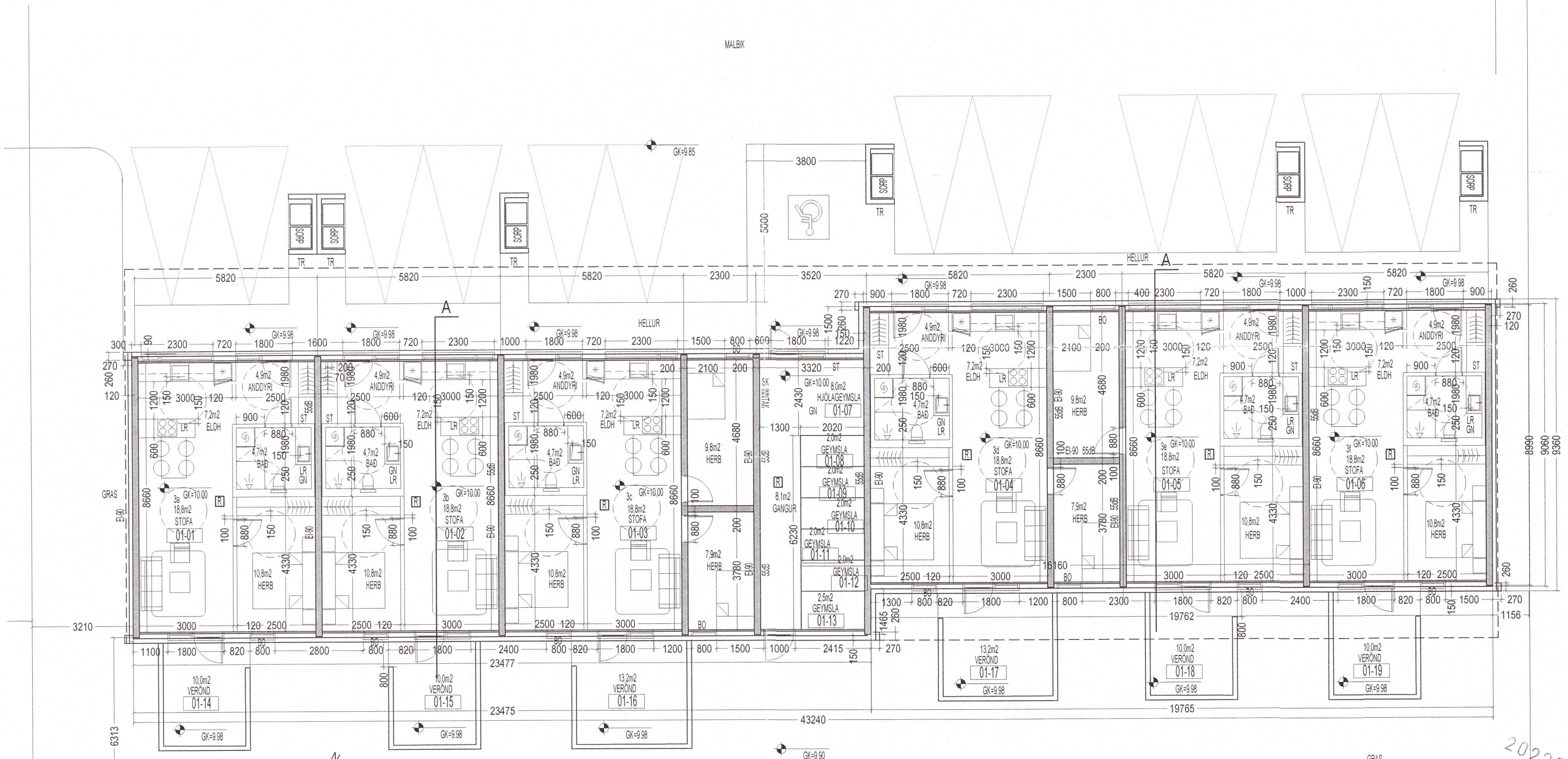
GRUNNMYND, MKV. 1:100
