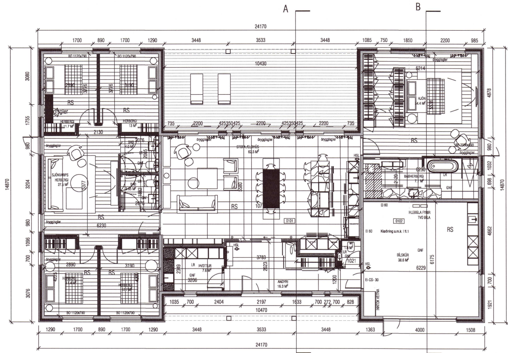
GRUNNMYND
