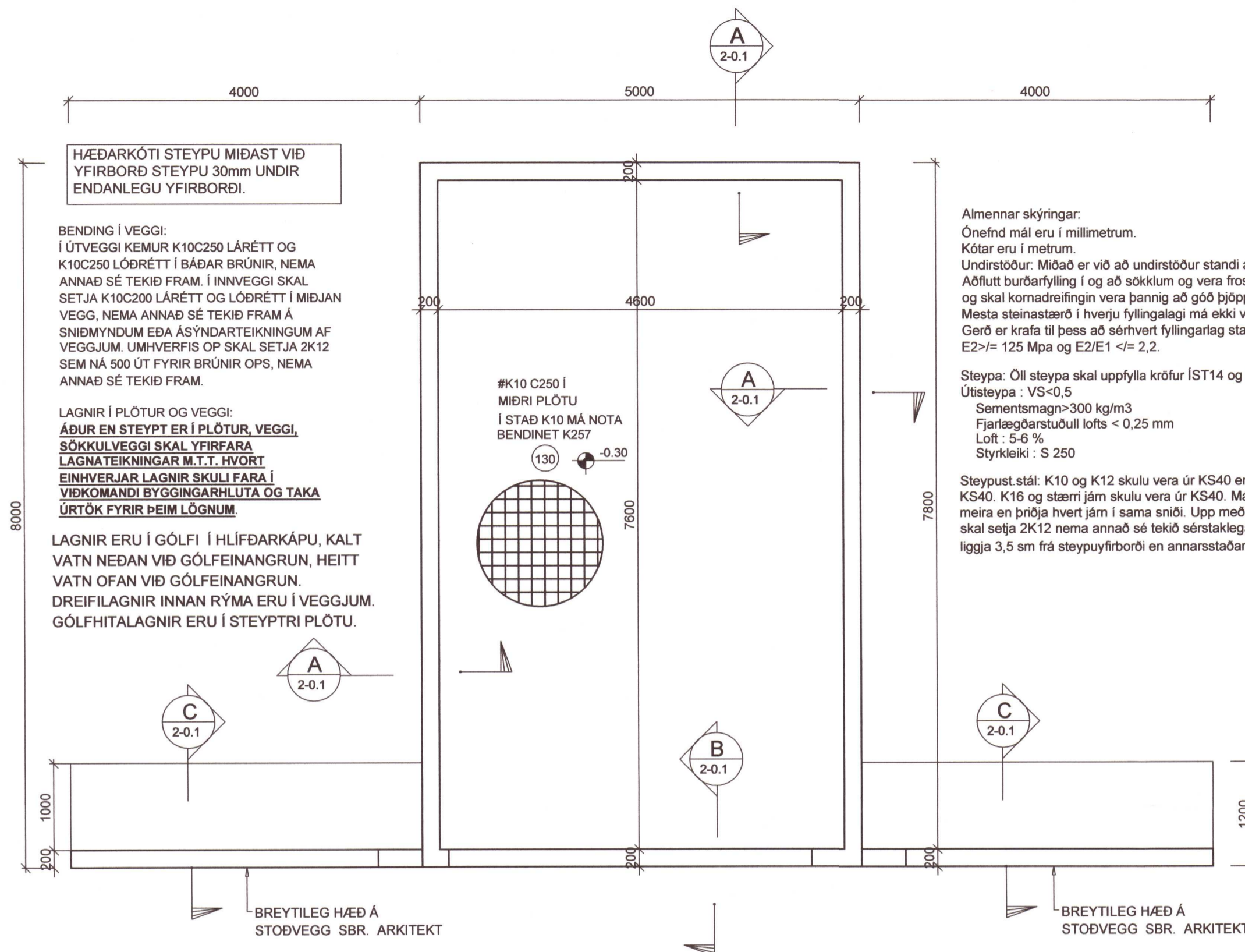
GRUNNMYND SÖKKLA 1:50
