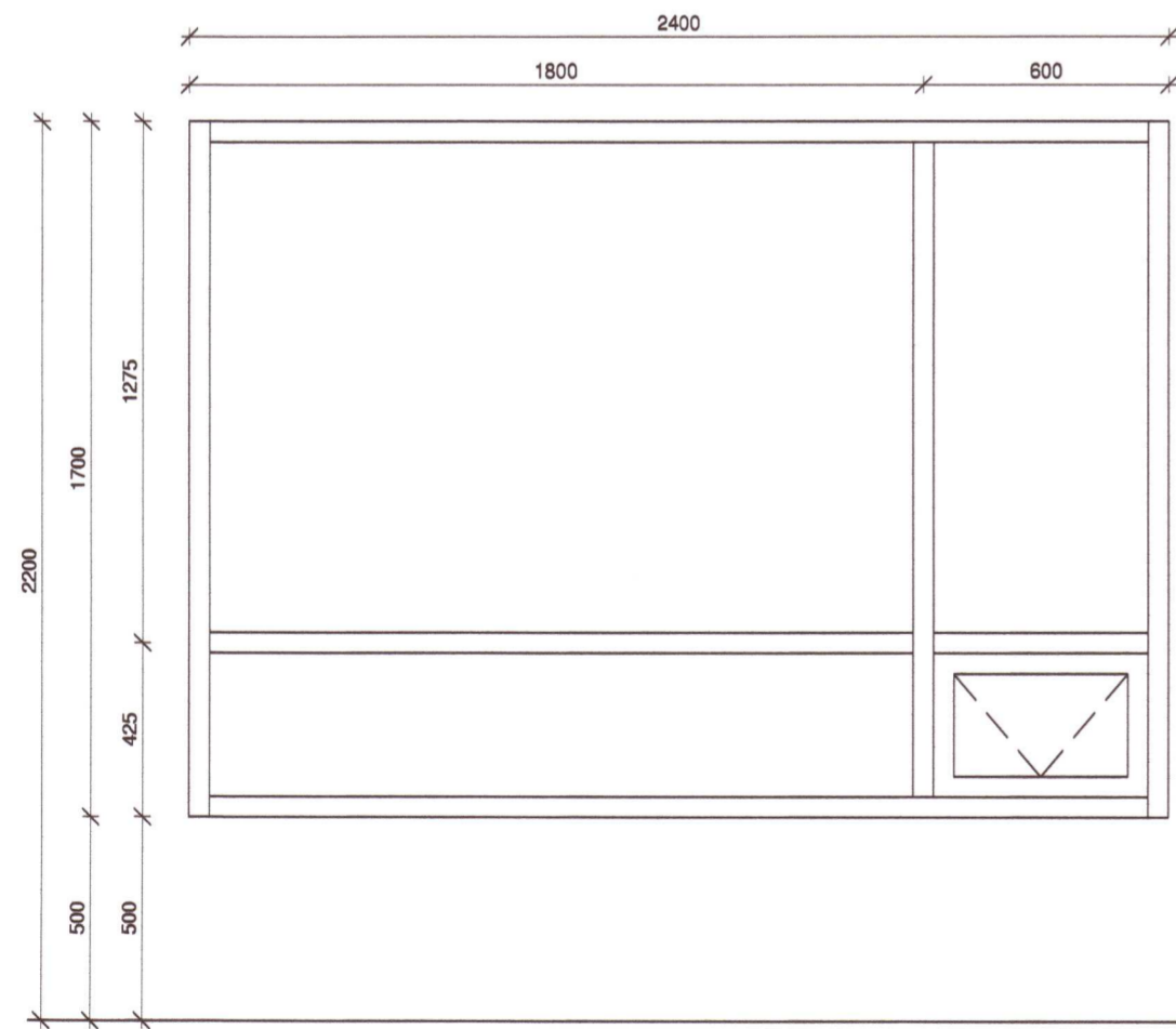
G6. Opnun á fagl..... Topphengt Fjöldi..... 1 stk
