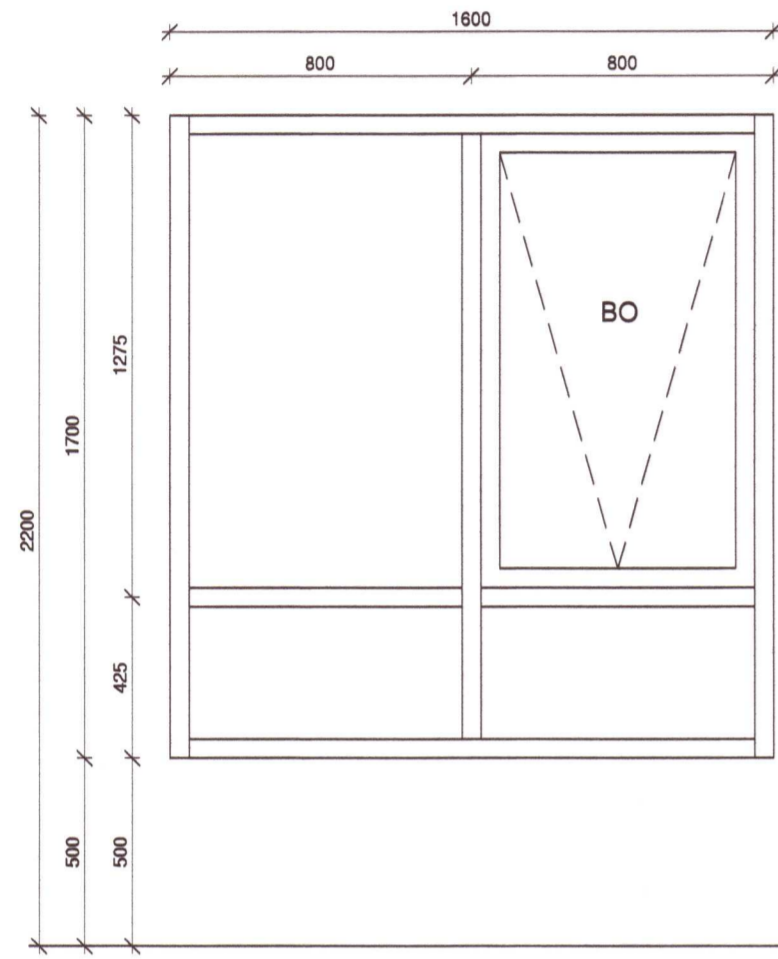
G1. Opnun á fagl..... Topphengt Fjöldi..... 2 stk
