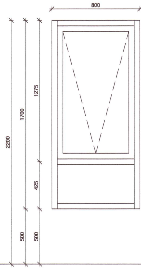
G2. Opnun á fagl..... Topphengt Fjöldi..... 2 stk
