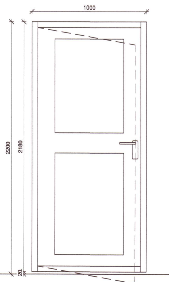
H1. Opnun á hurð..... Vinstri út Fjöldi..... 2 stk
