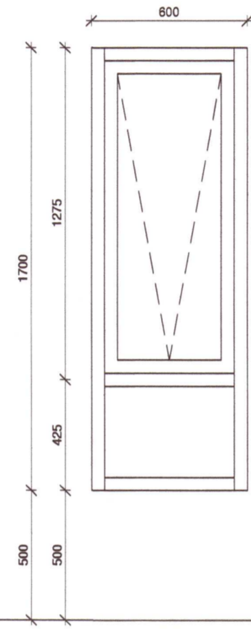
G3. Opnun á fagl..... Topphengt Fjöldi..... 2 stk
