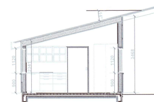
þversnið
