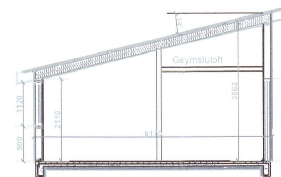
þversnið
